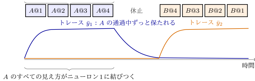
図 12.2: 動画が不変性をどう教えるか (模式図)。物体 A が四つの位置を通過し ( A@1 は位置 1 の A )、休息をはさんで物体 B が続く。 A の最初の見え方で勝ったニューロンのトレース (12.2) は通過の間ずっと保たれ、 A のすべての見え方が一つのニューロンに結びつく。休息がトレースを消し、 B は別のニューロンに割り当てられる。
