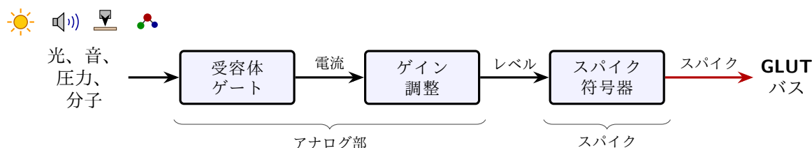
図 11.1: 変換の連鎖としての感覚器官。受容体タンパク質がチャンネルを開いて電流を生む。ゲイン調整がそれを状況に合わせる。符号器 (2.1) がレベルをスパイクに変え、スパイクは GLUT バスへ出ていく。目と耳では最初の段はスパイクをまったく出さない。遠くへ送る必要が生じるまで、信号はアナログのままである。
