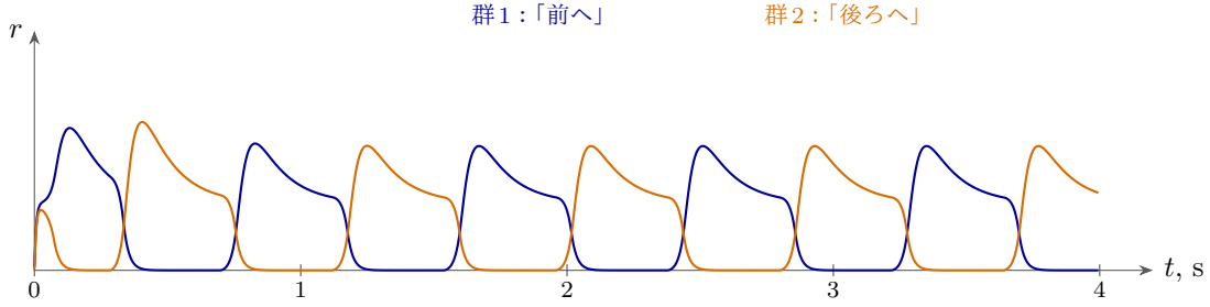
図 13.3: モデル (13.6) によるリズム発生器 : I = 1 , \beta = 2 , b = 2 , \tau = 20 ms, \tau_a = 0.4 s。相互抑制と疲労を持つ二つの群は、入力が一定の信号であるにもかかわらず、周期 0.84 s で交代に働く。
