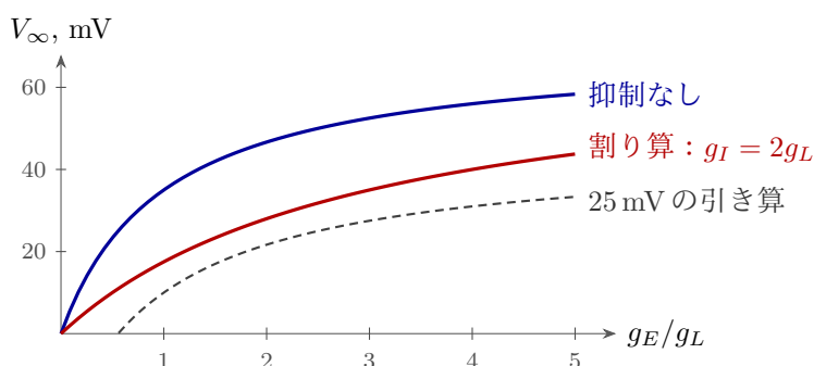
図 3.2: シャント抑制は電圧から引くのではなく、電圧を割る。青の曲線は抑制なしの定常電圧 (3.3)、赤は抑制性コンダクタンス g_I = 2g_L のあるもの。赤の曲線は青の曲線を横に3倍引き延ばしたものであり、入力を 1 + g_I/g_L = 3 で割ったのと同じである。破線は一定の25 mVを引く抑制で、曲線全体が下がり、傾きは変わらない。
