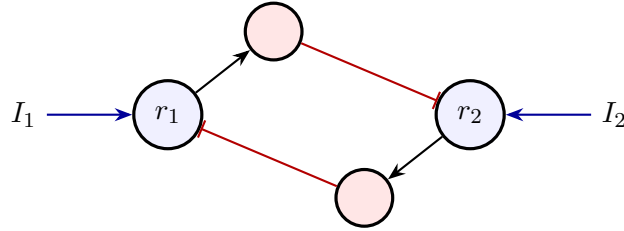
Рис. 3.3: Вибір із двох. Дві групи GLUT -нейронів (сині) гальмують одна одну через GABA -посередників (червоні).
