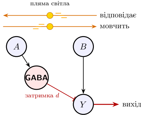
Рис. 3.1: Детектор напрямку руху. B збуджує Y , A гальмує його через GABA -посередника із затримкою d . За руху від A до B зі швидкістю близько \Delta x/d гальмування гасить збудження; за зворотного руху воно запізнюється. Жовта пляма з рисками — світло, що біжить над датчиками.
