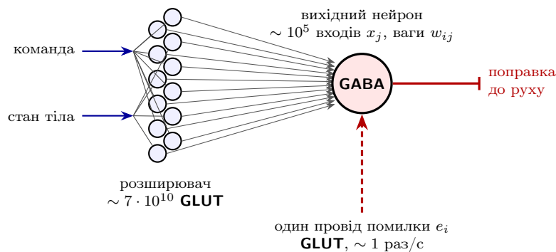
Рис. 15.1: Схема навчання з учителем, як її, схоже, реалізує мозок. Команда й стан тіла розкладаються величезним шаром GLUT-нейронів у довгий вектор x_j ; вихідний GABA-нейрон додає його з вагами w_{ij} . Єдиний провід помилки приносить e_i ; збіг помилки з активним входом послаблює вагу цього входу, як у правилі (15.1).
