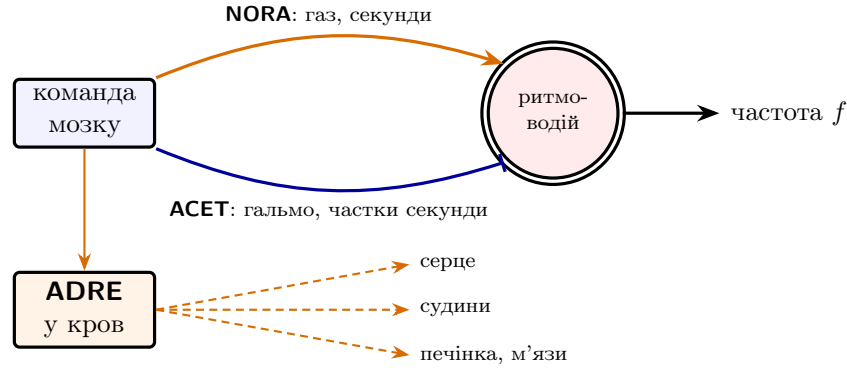
Рис. 16.1: Два проводи протилежного знака до ритмоводія серця: газ NORA повільний, гальмо АСЕТ швидке. Унизу — той самий газ широкомовною шиною: ADRE -клітини викидають адреналін у кров, і сигнал отримують усі органи з відповідним рецептором (штрихові стрілки).
