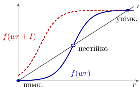
Рис. 2.5: Пам'ять із групи GLUT -нейронів із сильним зворотним зв'язком. Суцільна крива — без зовнішнього припливу: два стійкі перетини з прямою r , «вимкнено» й «увімкнено», і нестійкий між ними. Короткий приплив I (штрихова крива) залишає лише верхній.
