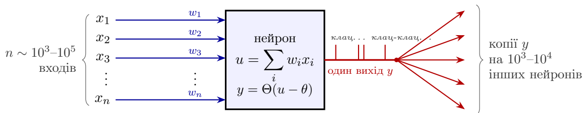
Рис. 1.1: Нейрон очима інженера. Багато входів x_i , кожен зі своєю вагою w_i ; усередині — зважена сума u і порівняння з порогом \theta ( \Theta — сходинка: 1, якщо аргумент додатний, і 0 інакше); один вихід y — послідовність імпульсів, розмножена розгалуженням на тисячі отримувачів.
