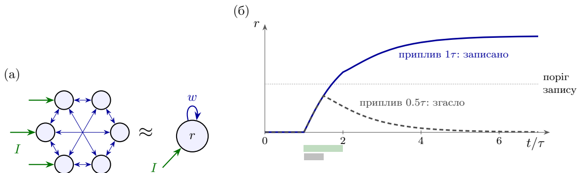
Рис. 2.4: Група, сильно зв'язана сама з собою. (а) Багато GLUT -нейронів, що збуджують одне одного, поведуться як один нейрон із частотою r , який збуджує сам себе із силою w ; ззовні надходить приплив I . (б) Частота групи в часі при w = 1 і тій самій кривій f , що на рис. 2.5. Приплив I = 0.6 подається на час, позначений смужкою під віссю. Якщо він триває 1\tau , група встигає перейти нестійку точку r = 0.5 , розгоряється й лишається горіти, коли приплив закінчився. Якщо лише 0.5\tau , вона не дотягує до цієї точки й згасає назад: щоб записати біт, приплив має тривати довше приблизно 0.7\tau .
