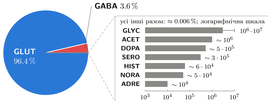
Рис. 1.2: Частки типів нейронів у мозку за оцінками таблиці 1.1. Коло майже цілком зайняте GLUT ; GABA — вузький сектор, а всі інші типи разом — волосина на межі. Праворуч цю волосину збільшено, за логарифмічною шкалою кількості нейронів; для GLYC стовпчик сягає середини діапазону 10^6 - 10^7 , відрізок показує весь діапазон. Для ASPA оцінки немає, і на рисунку його немає.
