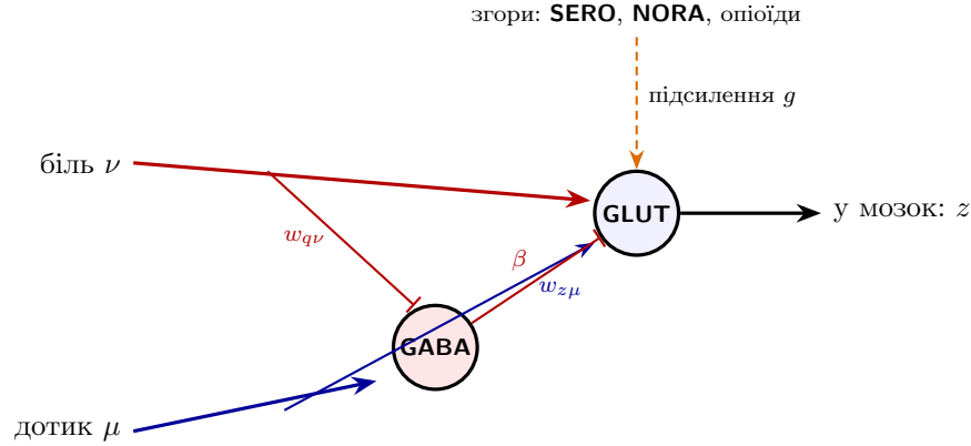
Рис. 14.1: Ворота болю в спинному мозку за моделлю (14.2). Вихідний GLUT -нейрон отримує біль \nu і слабке збудження від дотику \mu . Гальмівний посередник ( GABA або GLYC ) збуджується дотиком і, за припущенням теорії воріт, вимикається болем. Згори, широкомовними каналами, надходить підсилення g .
