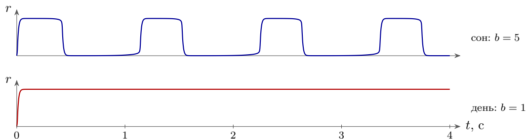
Рис. 20.2: Та сама група (20.2) у двох режимах: w = 5 , I = 2 , \theta = 2.5 , \tau = 10 мс, \tau_a = 0.3 с. Із сильною втомою ( b = 5 , як у повільному сні) група гойдається між роботою й тишею з періодом 1.1 с (значення моделі; у корі період більший за секунду, під наркозом — близько 3 с). Послабмо втому ( b = 1 ) — так діє ацетилхолін — і та сама група працює рівно.
