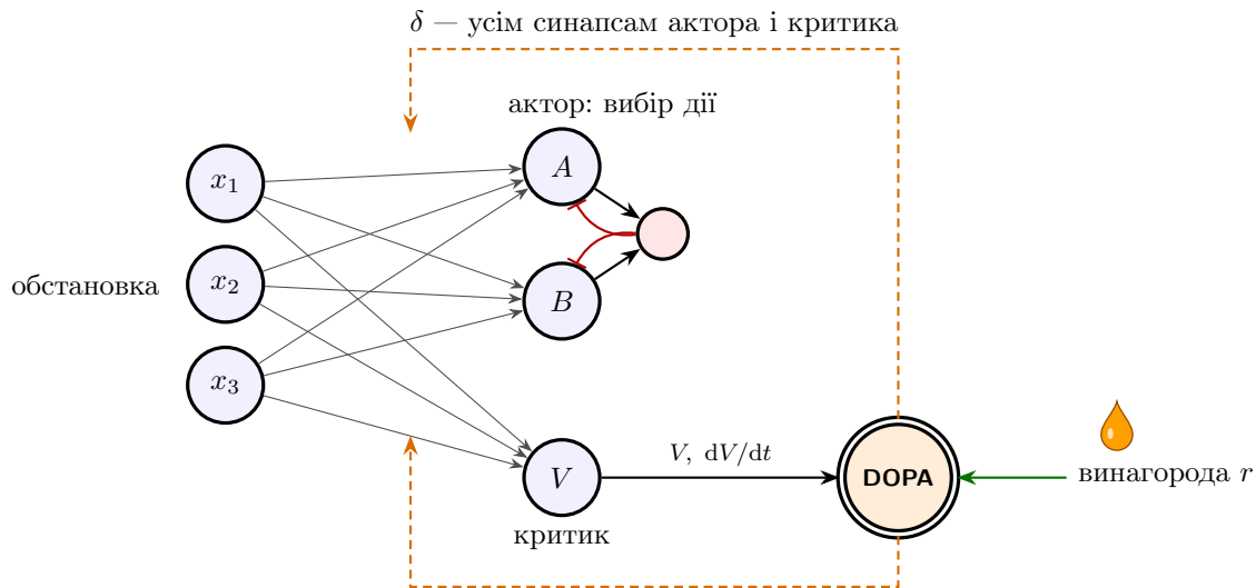
Рис. 6.5: Мережа, яка навчається вибирати дії. Сірі стрілки — GLUT -синапси зі змінними вагами; червоний кружок — GABA -нейрон; подвійний кружок — DOPA -ритмоводій, що обчислює \delta за (6.8); штрихові стрілки — широкомова розсилка \delta .
