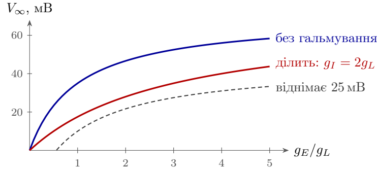
Рис. 3.2: Шунтувальне гальмування ділить напругу, а не віднімає від неї. Синя крива — усталена напруга (3.3) без гальмування, червона — з гальмівною провідністю g_I = 2g_L . Червона — та сама синя, розтягнута по горизонталі втричі: вхід ніби поділили на 1 + g_I/g_L = 3 . Штрихова — гальмування, що віднімає сталі 25 мВ: крива опускається цілком, нахил не змінюється.
