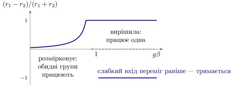
Рис. 8.2: Вибір із двох за різного коефіцієнта підсилення, входи відрізняються на \varepsilon = 0.05 . При g\beta > 1 стійкі обидва рішення (суцільні лінії; перемога слабого входу — при g\beta > (1 + \varepsilon)/(1 - \varepsilon) \approx 1.1 ), і мережа тримає те, яке вже ухвалила; симетричний стан (штрихова лінія) нестійкий.
