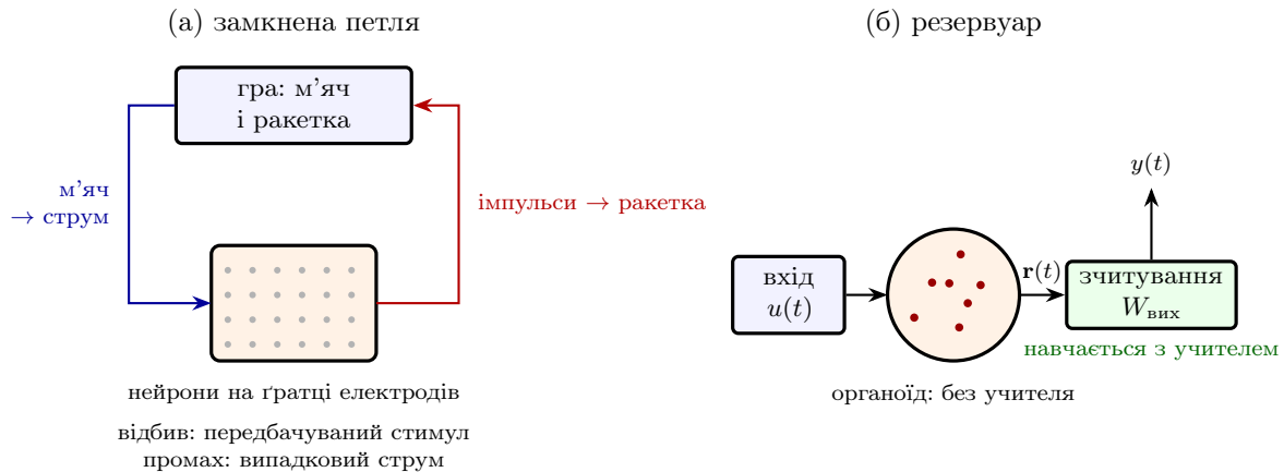
Рис. 21.1: Два способи змусити живу мережу обчислювати. (а) Замкнена петля: положення м'яча подається струмом, імпульси рухових ділянок рухають ракетку, а передбачуваний або випадковий стимул після удару слугує учителем. (б) Резервуар (21.2): організму не подають навчального сигналу, він розщеплює вхід на безліч нелінійних відгуків із пам'яттю; за помилкою навчається лише одне лінійне зчитування ззовні. Зв'язки самого організму при цьому теж змінюються — без учителя.
