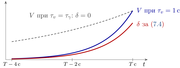
Рис. 7.2: Зростання дофаміну під час наближення до винагороди як помилка передбачення, \tau_\gamma = 4c . Штрихова лінія — очікування, що росте рівно так, як вимагає горизонт ( \delta = 0 ); синя — очікування, що росте крутіше; червона — помилка (7.4).
