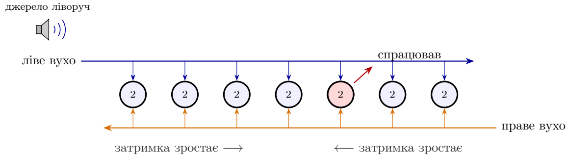
Рис. 2.3: Визначення напрямку на звук. Сигнали від двох вух біжать назустріч один одному; кожен кружечок — детектор збігів із порогом 2. Якщо звук прийшов у праве вухо пізніше, сигнали зустрічаються правіше від середини, за формулою (2.5). Вихід мережі — номер нейрона, що спрацював. Тут джерело ліворуч: у ліве вухо звук прийшов раніше.
