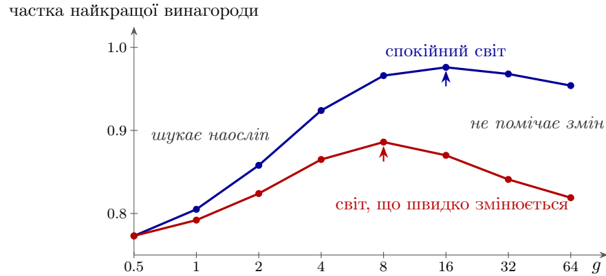
Рис. 8.3: Частка найкращої можливої винагороди за сталого коефіцієнта підсилення g (шкала за g логарифмічна). Синя крива — світ змінюється в середньому раз на тисячу спроб, червона — раз на двадцять. Стрілки позначають найкраще g : у світі, що швидко змінюється, воно вдвічі менше. Середнє за 60 прогонами по 4000 спроб.
