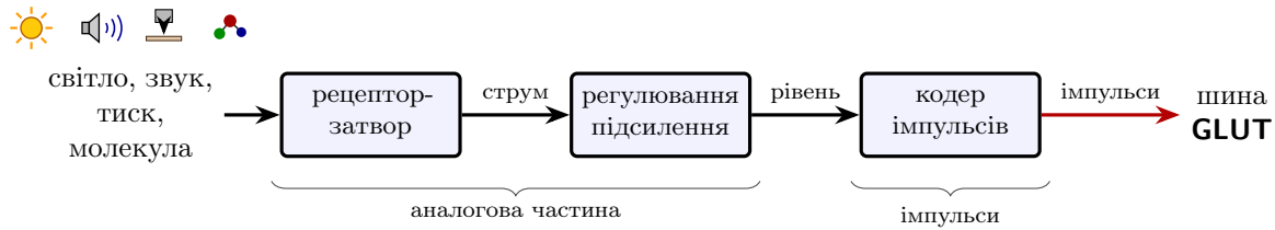
Рис. 11.1: Будь-який орган чуття як ланцюг перетворень. Білок-рецептор відкриває канал і дає струм; регулювання підсилення пристосовує його до обставин; кодер (2.1) перетворює рівень на імпульси, які йдуть на шину GLUT . В оці й вусі перші каскади взагалі не видають імпульсів: сигнал лишається аналоговим, доки не доводиться передавати його далеко.
