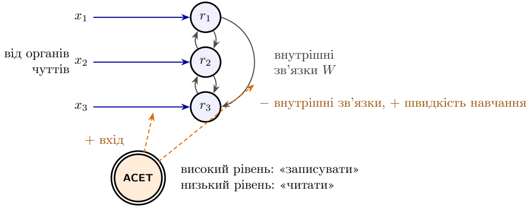
Рис. 9.1: АСЕТ як лінія дозволу запису. Нейрони r_i отримують вхід x_i від органів чуттів (сині стрілки) і збуджують один одного через внутрішні зв'язки W (сірі), у яких зберігаються образи. Ацетилхолін (штрихові стрілки) посилює вхід, послаблює внутрішні зв'язки і полегшує зміну ваг, як у (9.1).
