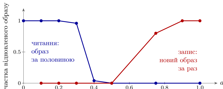
Рис. 9.2: Модель (9.1): 200 нейронів, образи по 20 активних, середнє за десятима прогонами. Сині точки — читання: яку частку образу відновлено за його половиною після того, як підказку прибрано. Червоні точки — запис: яка частка нового образу, наполовину схожого на старий, згадується після одного пред'явлення, якщо ацетилхолін задає і швидкість навчання. Читання працює при a \leq 0.3 , запис — при a \geq 0.9 .
