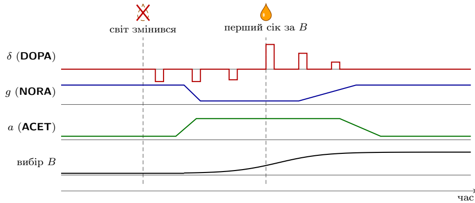
Рис. 10.2: Одна подія, простежена через усю машину. Це якісна схема за моделями й гіпотезами розділів 6–9, а не результат розрахунку. Після зміни DOPA відповідає провалами; повторні провали, за гіпотезою, піднімають сигнал несподіванки, NORA знижує підсилення, ACET вмикає запис; перший сік за B дає сплеск, вибір переходить на B , і ручки повертаються.
