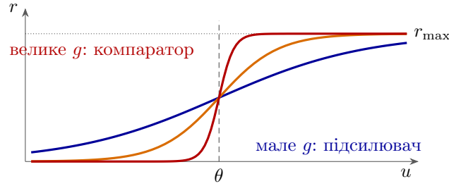
Рис. 8.1: Передавальна характеристика (8.1) за трьох значень коефіцієнта підсилення g .
