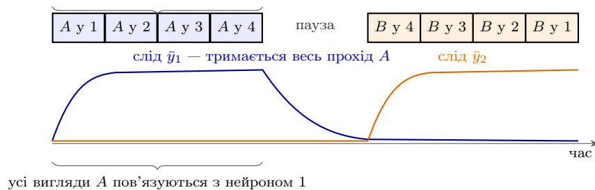
Рис. 12.2: Як відео навчає інваріантності, схема. Предмет A проходить через чотири положення, потім пауза, потім предмет B . Слід (12.2) нейрона, що виграв на першому вигляді A , тримається весь прохід, і всі вигляди A виявляються пов'язаними з одним нейроном. Пауза стирає слід, і B дістається іншому нейрону.
