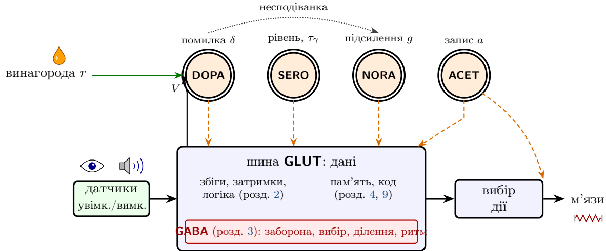
Рис. 10.1: Машина цілком. Шина GLUT несе дані від датчиків до вибору дії; GABA керує потоком усередині неї. Подвійні кружки — широкомовні канали; штрихові стрілки — розсилання їхніх сигналів усій мережі, у кожного своя ручка. DOPA отримує винагороду r і очікування V від критика всередині шини (розд. 6); точкова стрілка — гіпотеза, що про несподіванку NORA дізнається з незвично великих помилок (розд. 8).
