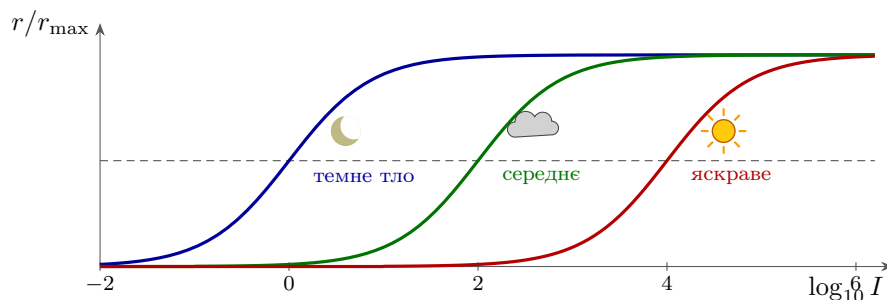
Рис. 11.2: Регулювання підсилення датчика світла за (11.2). Кожна крива охоплює два-три порядки яскравості; при переході на яскравіше тло \sigma зростає, і крива зсувається логарифмічною віссю. Разом криві, що зсуваються, покривають увесь діапазон.
