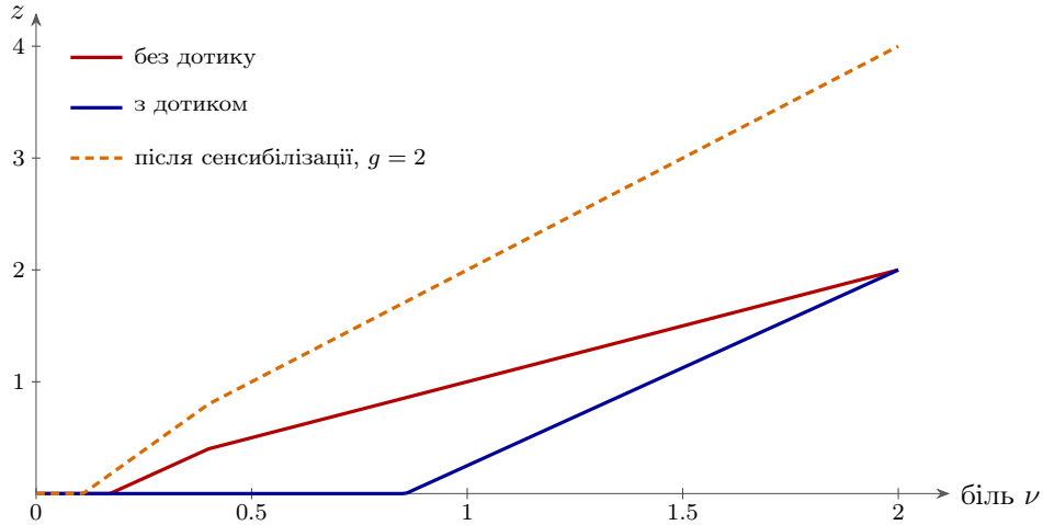
Рис. 14.2: Вихід воріт (14.2) залежно від сили болю. Дотик піднімає поріг і приглушує слабкий і середній біль, але не сильний. Сенсibiliзація (штрихова лінія) вдвічі збільшує підсилення: той самий біль передається вдвічі гучніше, а поріг опускається.
