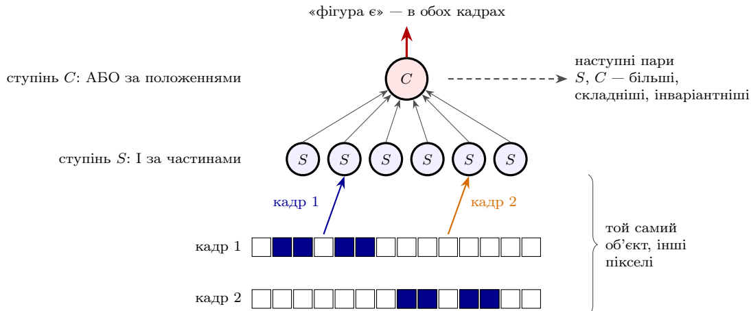
Рис. 12.1: Одна пара ступенів конвеєра. Нейрони S шукають те саме поєднання частин у різних місцях; нейрон C відповідає, якщо воно знайшлося хоч десь (12.1). Фігура в кадрі 1 і в кадрі 2 збуджує різні S -нейрони, але той самий C . Наступні пари ступенів повторюють те саме на дедалі більших і складніших поєднаннях.
