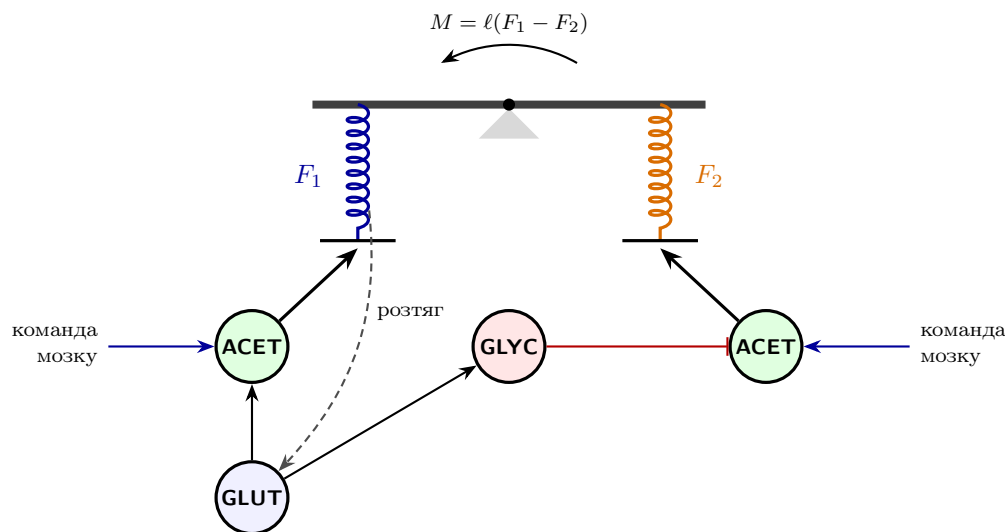
Рис. 13.2: Два м'язи на один суглоб і найшвидша петля зворотного зв'язку. ACET -нейрони отримують команди мозку й тягнуть суглоб у різні боки; різниця сил повертає його, сума робить жорсткішим. Датчик розтягу ( GLUT ) лівого м'яза збуджує його власний ACET -нейрон і через GLYC -посередника гальмує нейрон м'яза-антагоніста — заборона з розділу 3.
