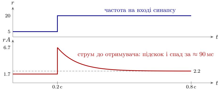
Рис. 4.4: Синапс, що виснажується, за формулою (4.6) при U = 0.5 , \tau_{\text{відн}} = 0.8 с; струм в одиницях A_0 за секунду, штрихова лінія — усталений струм: він зріс лише з 1.7 до 2.2, а в момент стрибка — до 6.7. Синапс повідомляє отримувачеві про те, що частота змінилася, а не про те, яка вона.
