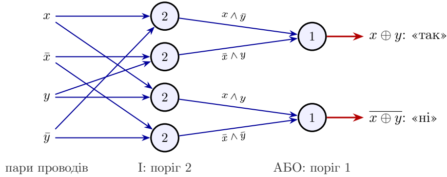
Рис. 2.2: Виключне АБО на двопровідному коді, лише з GLUT -нейронів. Число в кружечку — поріг в одиницях ваги одного входу. Чотири нейрони I впізнають чотири комбінації входів, два нейрони АБО збирають їх у пару проводів відповіді.
