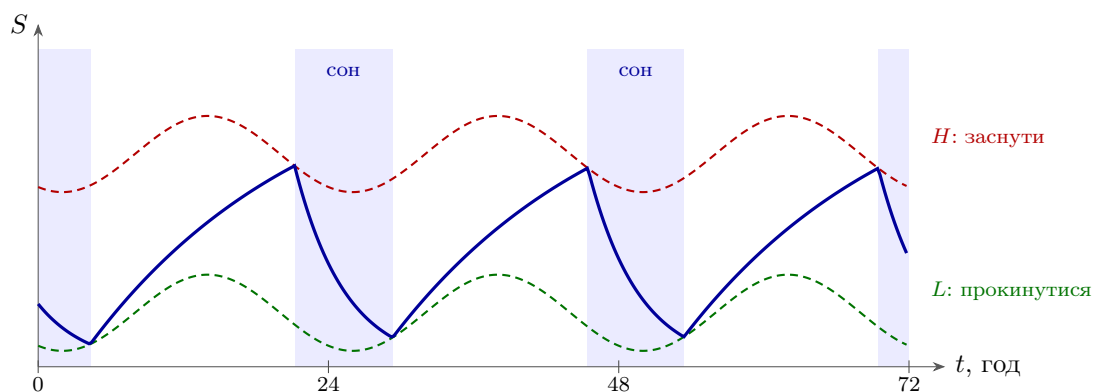
Рис. 20.1: Тиск сну S (20.1) за \tau_r = 18.2 год, \tau_d = 4.2 год. Удень S заряджається до верхнього порога H , уночі (зафарбовано) розряджається до нижнього L ; обидва пороги гойдаються разом із добовим ритмом. Машина сама приходить до режиму близько 16 годин неспання і 8 годин сну.
