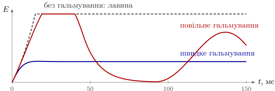
Рис. 3.4: Частота GLUT -групи зі зворотним зв'язком w_{EE} = 1.5 , \tau_E = 10 мс, після ввімкнення входу. Без гальмування (штрих) активність зростає без меж. З гальмуванням сили w_{EI}w_{IE} = 2 і \tau_I = 2 мс (синя крива) вона виходить на рівень E^* = h/(1 - 1.5 + 2) = 0.67h . З тим самим гальмуванням, але повільним, \tau_I = 30 мс (червона крива), активність коливається.
