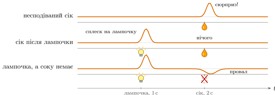
Рис. 1.4: Частота імпульсів DOPA-нейронів у трьох дослідних умовах (схематично, за [2]). Пунктир — рівня фонові частоти. Лампочка — сигнал, крапля — сік, перекреслена крапля — сік, який обіцяли, але не дали. Відгук — помилка передбачення (1.2).
