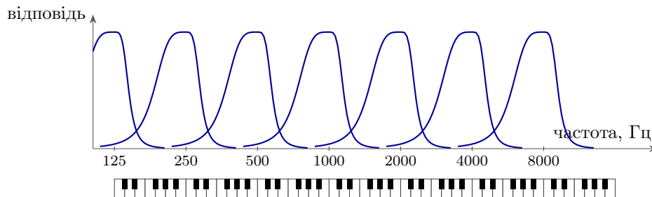
Рис. 11.3: Вуха як банк смугових фільтрів, схема. Кожна крива — відповідь датчиків однієї ділянки на звук різної частоти; центральні частоти йдуть через октаву, як клавіші на логарифмічній шкалі. У справжніх фільтрів крутий високочастотний схил і пологий низькочастотний. Унизу — клавіатура: на ній, як і у вусі, кожній октаві дістається однакове місце.
