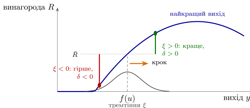
Рис. 6.3: Шум як пошук (6.6). Вихід нейрона тремтить навколо f(u) . Випадкове відхилення праворуч (зелене) дало більше за очікуване, \delta > 0 ; ліворуч (червоне) — менше, \delta < 0 . В обох випадках добуток \delta \xi додатний, і вага зсувається праворуч, туди, де винагорода росте. У середньому крок пропорційний нахилу R' : на вершині гірки відхилення в обидва боки однаково погані, і кроки гасять один одного.
