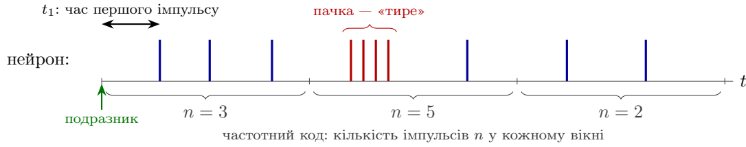
Рис. 4.1: Абетка Морзе й абетка нейрона. Ту саму послідовність імпульсів можна прочитати по-різному: порахувати імпульси у вікнах по 50 мс (підрозділ 4.4), виміряти затримку t_1 (4.4) або помітити пачку — «тире» (4.7).
