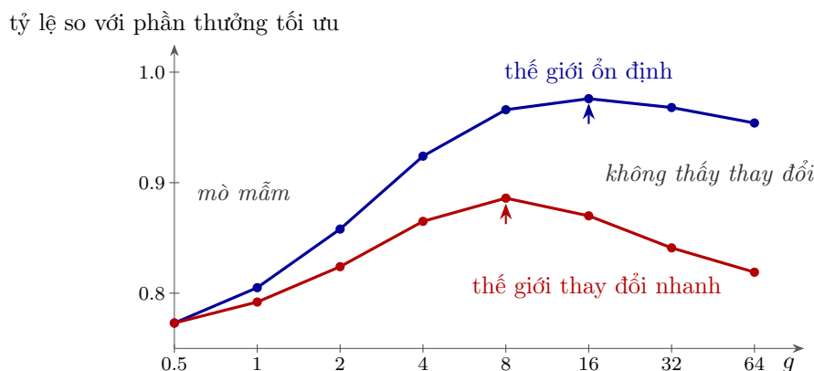
Hình 8.3: Tỷ lệ so với phần thưởng tốt nhất có thể khi hệ số khuếch đại g cố định (thang g là thang logarit). Đường xanh: thế giới thay đổi trung bình một lần sau mỗi nghìn lượt thử; đường đỏ: một lần sau mỗi hai mươi lượt. Mũi tên đánh dấu g tốt nhất: trong thế giới thay đổi nhanh, nó chỉ bằng một nửa. Trung bình của 60 lần chạy, mỗi lần 4000 lượt thử.
