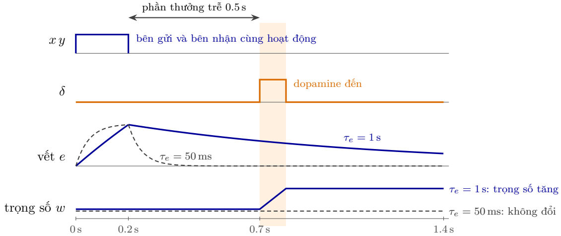
Hình 6.2: Vết theo quy tắc (6.5). Hoạt động đồng thời kéo dài 0.2s, dopamine đến nửa giây sau khi nó kết thúc. Các vết được vẽ theo tỷ lệ với giá trị cực đại của chính nó. Vết chậm ( \tau_e = 1 s) lúc đó vẫn còn, vết nhanh ( \tau_e = 50 ms) đã tan từ lâu.
