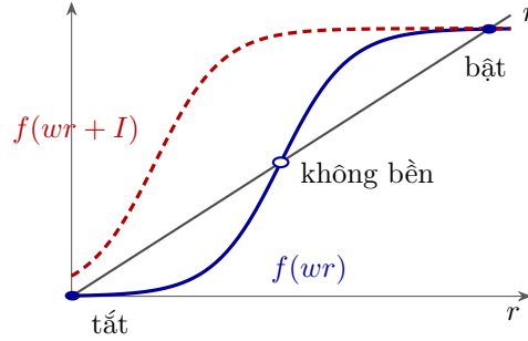
Hình 2.5: Bộ nhớ từ một nhóm nơ-ron GLUT có hồi tiếp mạnh. Đường liền là khi không có dòng vào từ bên ngoài: hai giao điểm bền với đường thẳng r , “tắt” và “bật”, và một giao điểm không bền ở giữa. Một dòng vào ngắn I (đường nét đứt) chỉ để lại giao điểm trên.
