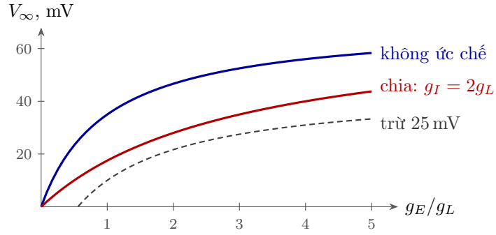
Hình 3.2: Ước chế sun chia điện áp chứ không trừ khỏi nó. Đường xanh là điện áp xác lập (3.3) khi không có ức chế, đường đỏ là khi có độ dẫn ức chế g_I = 2g_L . Đường đỏ chính là đường xanh bị kéo giãn gấp ba theo chiều ngang: như thể đầu vào bị chia cho 1 + g_I/g_L = 3 . Đường nét đứt là ước chế trừ đi một lượng không đổi 25 mV: cả đường cong hạ xuống, độ dốc không đổi.
