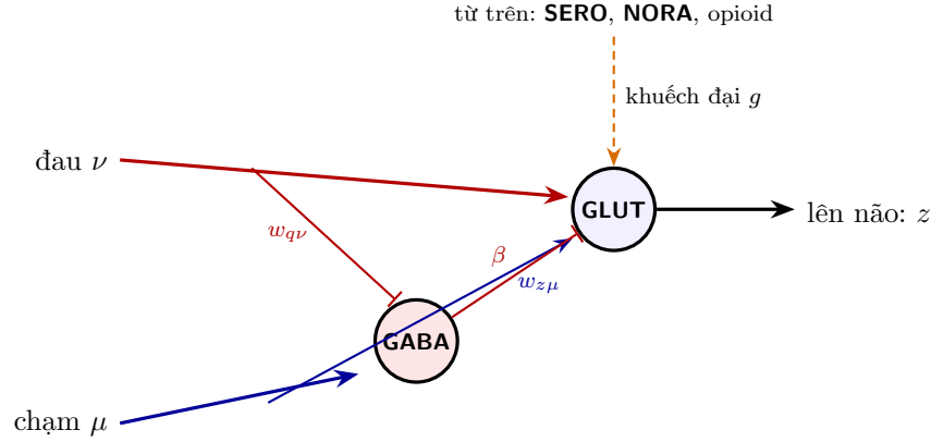
Hình 14.1: Cổng đau trong tủy sống theo mô hình (14.2). Nơ-ron GLUT đầu ra nhận cơn đau \nu và kích thích yếu từ cái chạm \mu . Nơ-ron trung gian ức chế ( GABA hoặc GLYC ) được cái chạm kích thích và, theo giả định của thuyết cổng, bị cơn đau tắt đi. Từ trên, qua các kênh quảng bá, đến hệ số khuếch đại g .
