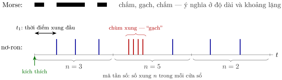
Hình 4.1: Mã Morse và mã của nơ-ron. Cùng một chuỗi xung có thể đọc theo nhiều cách: đếm số xung trong các cửa sổ 50 ms (mục 4.4), đo độ trễ t_1 (4.4), hoặc nhận ra một chùm xung — “gạch” (4.7).
