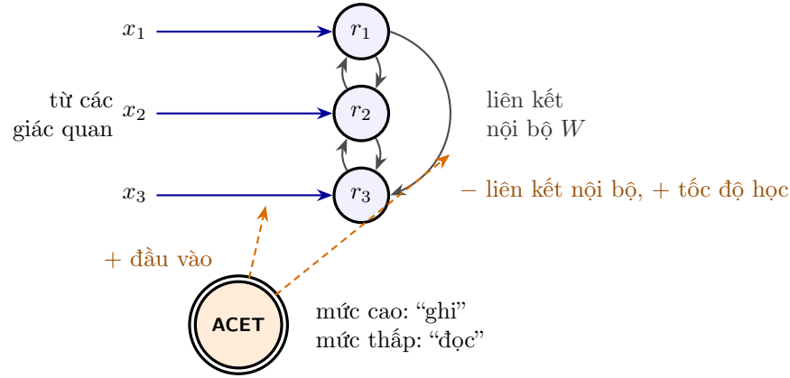
Hình 9.1: ACET là đường cho phép ghi. Các nơ-ron r_i nhận đầu vào x_i từ các giác quan (mũi tên xanh) và kích thích lẫn nhau qua các liên kết nội bộ W (màu xám), nơi lưu các mẫu. Acetylcholine (mũi tên nét đứt) tăng cường đầu vào, làm yếu liên kết nội bộ và làm trọng số dễ thay đổi hơn, như trong (9.1).
