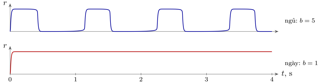
Hình 20.2: Cùng một nhóm (20.2) ở hai chế độ: w = 5 , I = 2 , \theta = 2.5 , \tau = 10 ms, \tau_a = 0.3 s. Với một mỗi mạnh ( b = 5 , như trong giấc ngủ sóng chậm), nhóm dao động giữa làm việc và im lặng với chu kỳ 1.1 s (giá trị của mô hình; trong vỏ não chu kỳ dài hơn một giây, khi gây mê khoảng 3 s). Làm yếu sự mệt mỗi ( b = 1 ), đúng như tác dụng của acetylcholine, và cùng nhóm ấy làm việc đều đặn.
