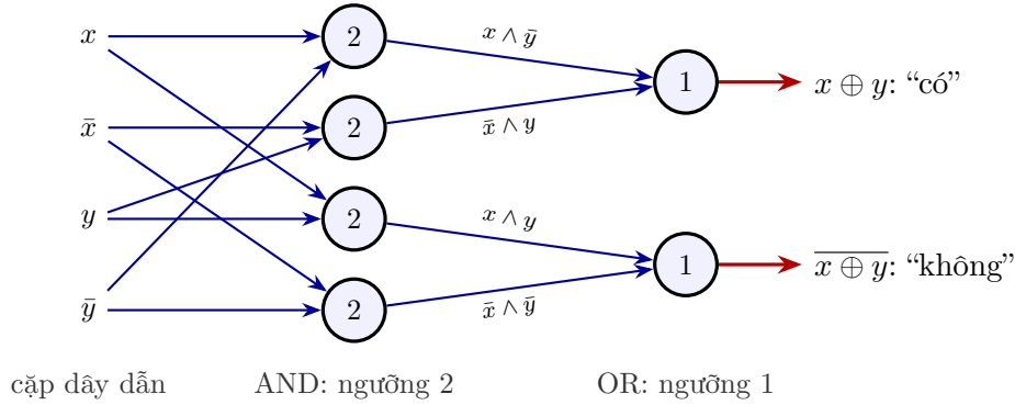
Hình 2.2: XOR trên mã hai dây, chỉ gồm các nơ-ron GLUT . Số trong vòng tròn là ngưỡng, tính theo đơn vị trọng số của một đầu vào. Bốn nơ-ron AND nhận ra bốn tổ hợp đầu vào, hai nơ-ron OR gom chúng thành cặp dây kết quả.
