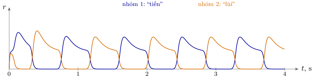
Hình 13.3: Bộ tạo nhịp theo mô hình (13.6): I = 1 , \beta = 2 , b = 2 , \tau = 20 ms, \tau_a = 0.4 s. Hai nhóm ức chế lẫn nhau và mỗi dần làm việc luân phiên với chu kỳ 0.84 s, dù tín hiệu đầu vào là không đổi.
