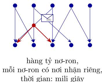
Hình 1.3: Hai cách truyền tin. Bên trái là bus địa chỉ, giống bưu điện với địa chỉ ghi trên phong bì; màu đỏ đánh dấu một nơ-ron và hai nơi nhận của nó. Bên phải là bus quảng bá, giống một đài phát thanh: một nhóm nhỏ nơ-ron nguồn, và mọi nơi đều nhận cùng một thông điệp.
