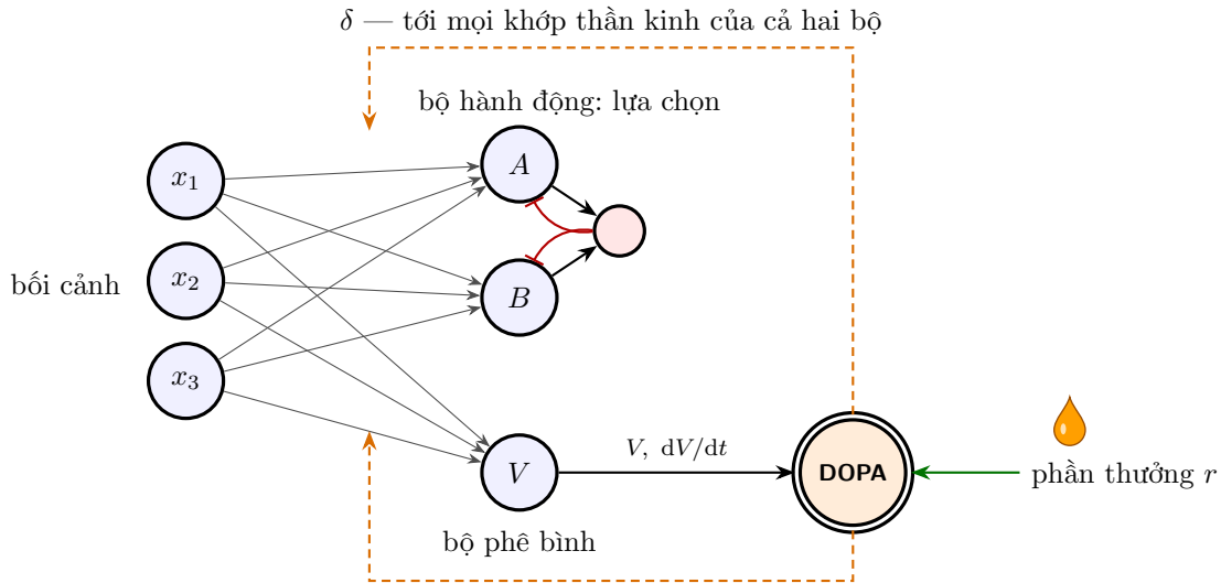
Hình 6.5: Mạng học cách chọn hành động. Mũi tên xám là các khớp thần kinh GLUT với trọng số thay đổi được; vòng tròn đỏ là nơ-ron GABA ; vòng tròn kép là bộ tạo nhịp DOPA , tính \delta theo (6.8); mũi tên nét đứt là việc phát quang bá \delta .
