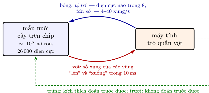
Hình 22.1: Vòng lặp DishBrain. Mũi tên xanh lam là đầu vào: vị trí bóng được ghi bằng mã vị trí và mã tần số (chương 4). Mũi tên đỏ là đầu ra: hiệu số đếm của hai vùng đẩy vợt. Đường nét đứt xanh lục là phản hồi sau mỗi lượt đánh, “thầy dạy” duy nhất của bàn thử.
