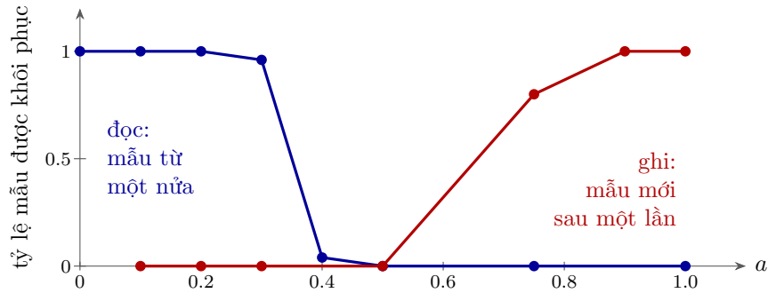
Hình 9.2: Mô hình (9.1): 200 nơ-ron, mỗi mẫu 20 nơ-ron hoạt động, trung bình qua mười lần chạy. Các điểm xanh là đọc: tỷ lệ mẫu được khôi phục từ một nửa của nó sau khi bỏ gợi ý. Các điểm đỏ là ghi: tỷ lệ của mẫu mới, giống một nửa với mẫu cũ, được nhớ lại sau một lần trình bày, nếu acetylcholine đặt cả tốc độ học. Đọc hoạt động khi a \leq 0.3 , ghi — khi a \geq 0.9 .
