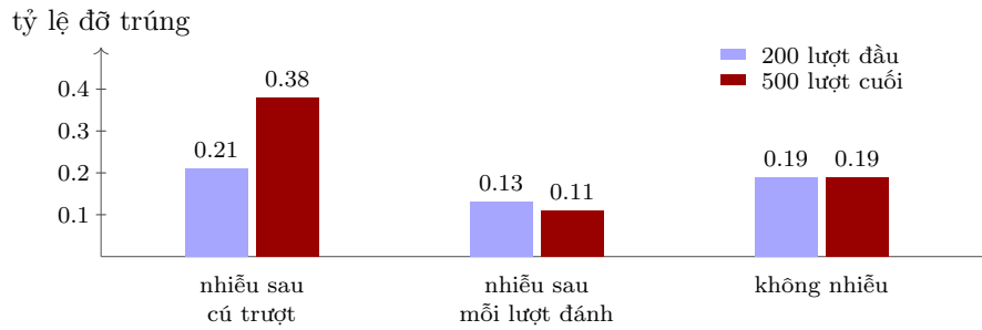
Hình 22.2: Mô hình “xáo trộn khi trượt” ( dishbrain_model.py ): tỷ lệ bóng đố trúng ở đầu và cuối 2000 lượt đánh, trung bình trên bốn mươi mô hình mẫu nuôi cấy. Việc học chỉ diễn ra nếu cú hích đi sau cú trượt chứ không đi sau cú trúng, cũng như trong thí nghiệm, nơi mức tăng có ý nghĩa trong một phiên chỉ có khi phản hồi đầy đủ.
