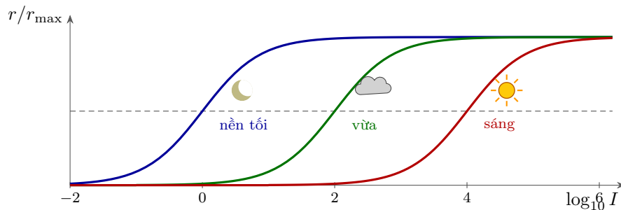
Hình 11.2: Điều chỉnh khuếch đại của cảm biến ánh sáng theo (11.2). Mỗi đường cong bao hai đến ba bậc độ sáng; khi chuyển sang nền sáng hơn, \sigma tăng và đường cong dịch theo trục logarit. Các đường cong dịch chuyển cùng nhau phủ kín toàn bộ dải.
