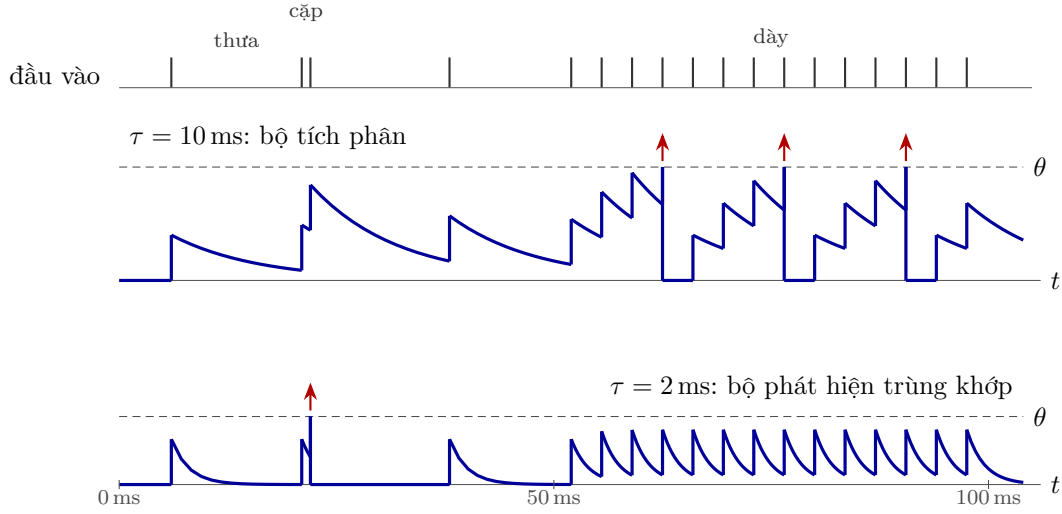
Hình 4.3: Cùng một đầu vào — hai nơi nhận khác nhau. Mỗi xung nâng điện áp thêm w , sau đó điện áp rò đi, như trong mô hình nơ-ron (2.1); mũi tên đỏ là xung của nơi nhận. Nơi nhận chậm ( \tau = 10 ms, \theta = 2.5w ) phát xung ở chỗ có nhiều xung và không nhận ra cặp xung. Nơi nhận nhanh ( \tau = 2 ms, \theta = 1.5w ) chỉ phát xung với cặp xung trong phạm vi cửa sổ (2.2), và bỏ qua dòng xung dày nhưng không trùng khớp.
