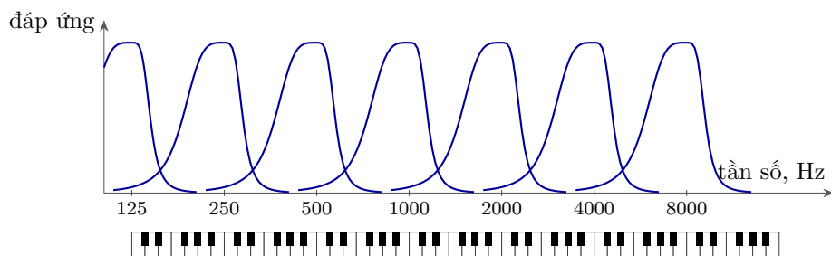
Hình 11.3: Tai như một dãy bộ lọc thông dải, sơ đồ. Mỗi đường cong là đáp ứng của các cảm biến trên một đoạn với âm có tần số khác nhau; các tần số trung tâm cách nhau một quãng tám, như phím đàn trên thang logarit. Bộ lọc thật có sườn tần số cao dốc và sườn tần số thấp thoải. Phía dưới là bàn phím: trên đó, cũng như trong tai, mỗi quãng tám chiếm chỗ như nhau.
