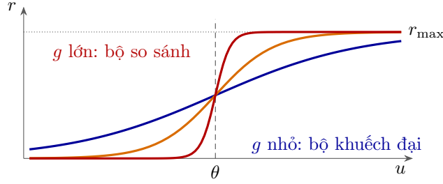
Hình 8.1: Đặc tuyến truyền đạt (8.1) với ba giá trị của hệ số khuếch đại g .
