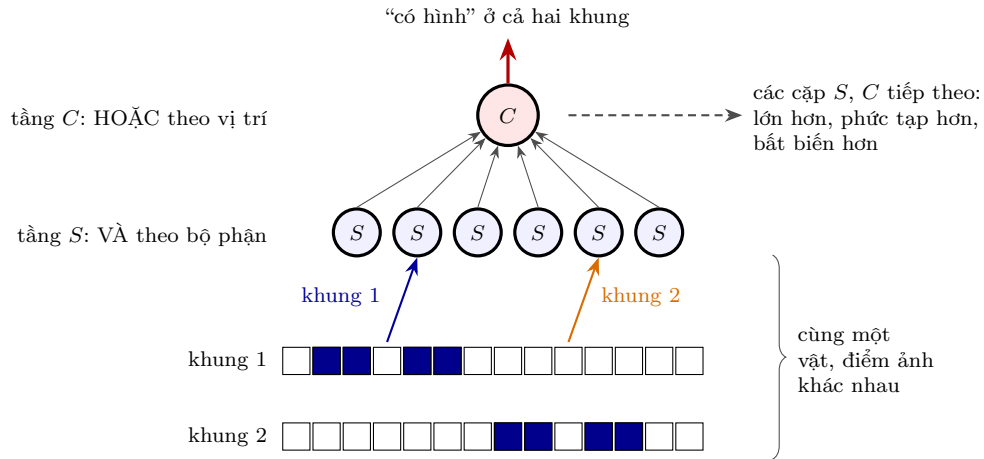
Hình 12.1: Một cặp tầng của dây chuyền. Các nơ-ron S tìm cùng một tổ hợp bộ phận ở những vị trí khác nhau; nơ-ron C đáp ứng nếu tổ hợp đó có ở bất cứ đâu (12.1). Hình ở khung 1 và ở khung 2 kích thích các nơ-ron S khác nhau, nhưng cùng một nơ-ron C . Các cặp tầng tiếp theo lặp lại điều đó với những tổ hợp ngày càng lớn và phức tạp.
