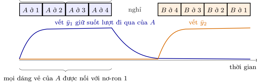
Hình 12.2: Video dạy tính bất biến như thế nào, sơ đồ. Đồ vật A đi qua bốn vị trí, sau đó là quãng nghỉ, rồi đến đồ vật B . Vết (12.2) của nơ-ron thắng ở dáng vẽ đầu tiên của A được giữ suốt lượt đi qua, và mọi dáng vẽ của A đều được nối với cùng một nơ-ron. Quãng nghỉ xóa vết, và B thuộc về một nơ-ron khác.
