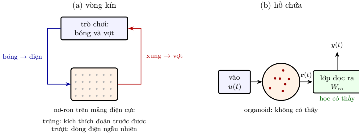
Hình 21.1: Hai cách buộc mạng sống tính toán. (a) Vòng kín: vị trí bóng được đưa vào bằng dòng điện, xung của các vùng vận động đẩy vợt, còn kích thích đoán trước được hoặc ngẫu nhiên sau cú đánh đóng vai thầy dạy. (b) Hồ chứa (21.2): organoid không nhận tín hiệu dạy nào, nó tách đầu vào thành nhiều đáp ứng phi tuyến có trí nhớ; chỉ một lớp đọc ra tuyến tính bên ngoài học theo sai số. Trong lúc đó, liên kết của chính organoid cũng thay đổi, không cần thầy.
