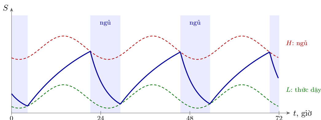
Hình 20.1: Áp lực ngủ S (20.1) với \tau_r = 18.2 giờ, \tau_d = 4.2 giờ. Ban ngày S nạp tới ngưỡng trên H , ban đêm (vùng tô màu) phóng xuống ngưỡng dưới L ; cả hai ngưỡng dao động theo nhịp ngày đêm. Cỗ máy tự đi tới chế độ khoảng 16 giờ thức và 8 giờ ngủ.
