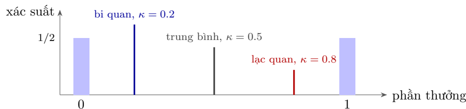
Hình 7.1: Phân bố phần thưởng được ghi lại bởi một tập nơ-ron DOPA . Phần thưởng bằng 0 hoặc 1 với xác suất 1/2 (các cột xanh); nơ-ron có tỷ lệ \kappa đi tới ước lượng V = \kappa (7.2).
