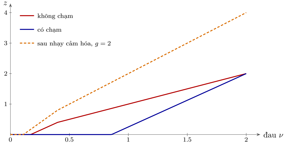
Hình 14.2: Đầu ra của cổng (14.2) theo cường độ đau. Cái chạm nâng ngưỡng và làm dịu cơn đau nhẹ và vừa, nhưng không làm dịu cơn đau mạnh. Nhảy cảm hóa (đường nét đứt) tăng hệ số khuếch đại gấp đôi: cùng một cơn đau được truyền to gấp đôi, còn ngưỡng hạ xuống.
