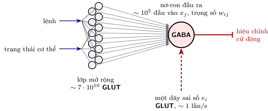
Hình 15.1: Sơ đồ học có giám sát, theo cách mà não dường như hiện thực. Lệnh và trạng thái cơ thể được một lớp khổng lồ các nơ-ron GLUT trải thành một vectơ dài x_j ; nơ-ron GABA đầu ra cộng nó với các trọng số w_{ij} . Dây sai số duy nhất mang e_i tới; sự trùng khớp giữa sai số và một đầu vào đang hoạt động làm yếu trọng số của đầu vào đó, như trong quy tắc (15.1).
