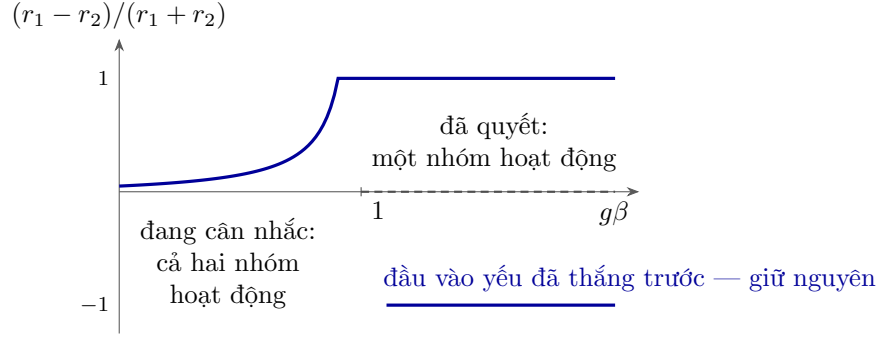
Hình 8.2: Lựa chọn giữa hai phương án với các hệ số khuếch đại khác nhau, các đầu vào khác nhau \varepsilon = 0.05 . Khi g\beta > 1 , cả hai lời giải đều ổn định (đường liền; đầu vào yếu thắng khi g\beta > (1 + \varepsilon)/(1 - \varepsilon) \approx 1.1 ), và mạng giữ lời giải nó đã chọn; trạng thái đối xứng (đường nét đứt) không ổn định.
