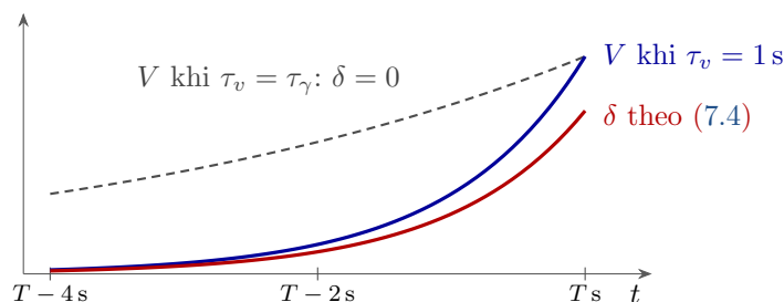
Hình 7.2: Dopamine tăng dần khi tiến gần phần thưởng, xem như sai số dự đoán, \tau_\gamma = 4 s. Đường nét đứt là kỳ vọng tăng đúng như tầm nhìn đòi hỏi ( \delta = 0 ); đường xanh là kỳ vọng tăng dốc hơn; đường đỏ là sai số (7.4).
