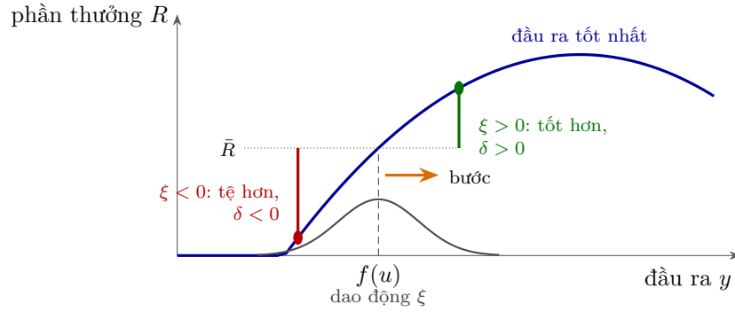
Hình 6.3: Nhiều là sự tìm kiếm (6.6). Đầu ra của nơ-ron dao động quanh f(u) . Độ lệch ngẫu nhiên sang phải (màu xanh lá) cho nhiều hơn kỳ vọng, \delta > 0 ; sang trái (màu đỏ) cho ít hơn, \delta < 0 . Trong cả hai trường hợp tích \delta \xi đều dương, và trọng số dịch sang phải, về phía phần thưởng tăng. Trung bình, bước tỷ lệ với độ dốc R' : trên đỉnh đồi, độ lệch về cả hai phía đều tệ như nhau, và các bước triệt tiêu lẫn nhau.
