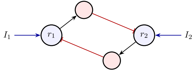
Hình 3.3: Chọn một trong hai. Hai nhóm nơ-ron GLUT (màu xanh) ức chế lẫn nhau qua các trung gian GABA (màu đỏ).
