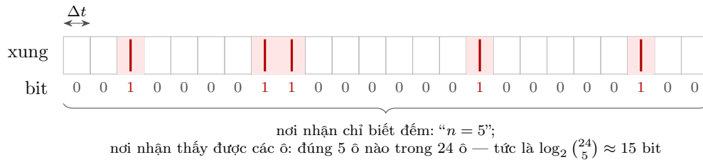
Hình 4.2: Dung lượng (4.1) đến từ đâu. Thời gian được cắt thành các ô dài \Delta t , trong mỗi ô hoặc có xung (1), hoặc không (0): dòng xung là một chuỗi nhị phân. Xung rơi vào một ô với xác suất p = r\Delta t . Ô càng nhỏ, chuỗi càng dài và càng nhiều bit; bộ đếm xung đánh mất gần như mọi thứ được ghi ở chỗ các số một nằm ở đâu.
