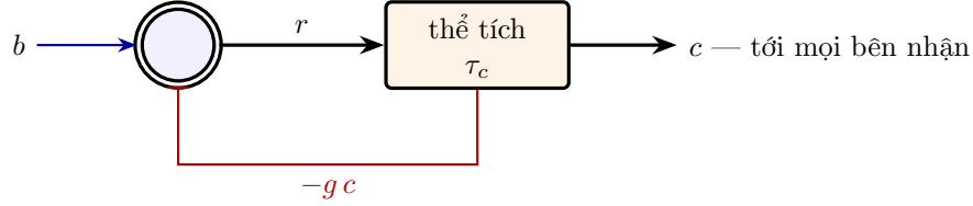
Hình 5.2: Nơ-ron SERO có hồi tiếp qua chính chất dẫn truyền của nó: nồng độ c đi tới mọi bên nhận và ức chế chính nơ-ron đó. Trong mô hình, đây là bộ điều chỉnh mức; vai trò như vậy của vòng lặp trong não là giả thuyết.
