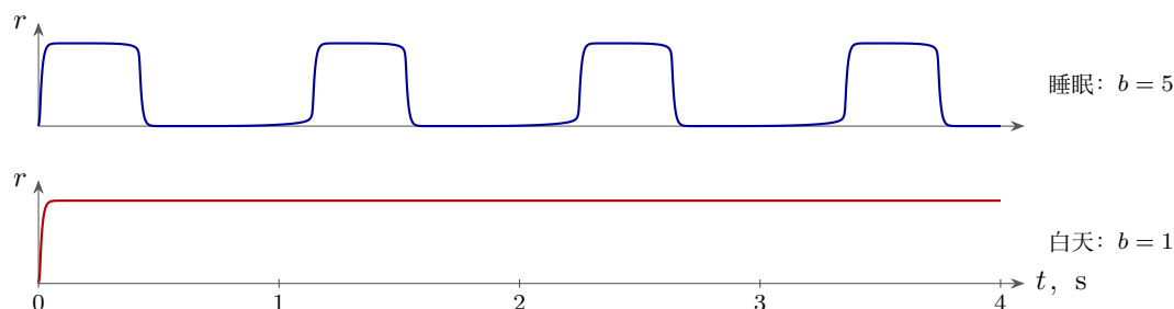
图 20.2: 同一个群体 (20.2) 在两种模式下: w = 5 , I = 2 , \theta = 2.5 , \tau = 10 ms, \tau_a = 0.3 s。疲劳强时 ( b = 5 , 如同慢波睡眠), 群体在工作与静默之间摆动, 周期为 1.1 s (模型值; 皮层中周期超过一秒, 麻醉下约为 3 s)。减弱疲劳 ( b = 1 ) —— 乙酰胆碱就是这样起作用的——同一个群体便平稳地工作。
