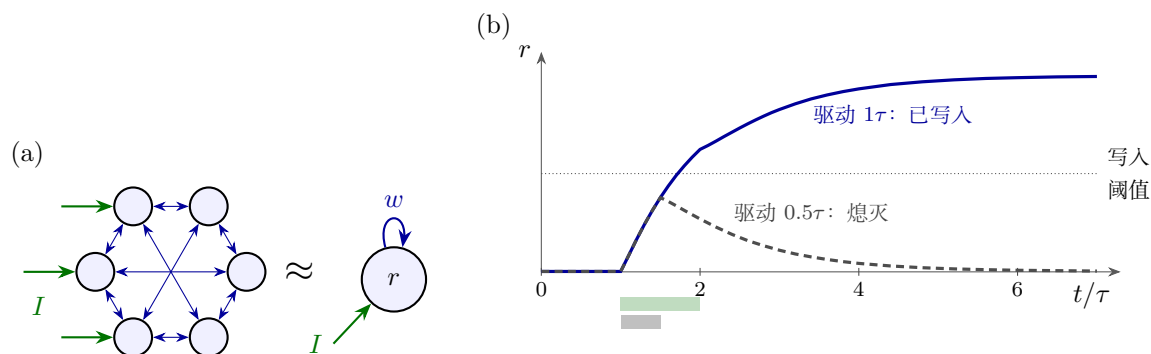
图 2.4: 与自身强连接的神经元群。(a) 许多相互兴奋的 GLUT 神经元，表现得就像一个频率为 r 、以强度 w 自我兴奋 of 的神经元；外部送来驱动 I 。(b) w = 1 、曲线 f 与图 2.5 相同时，神经元群的频率随时间的变化。驱动 I = 0.6 施加的时段用坐标轴下方的色条标出。如果它持续 1\tau ，神经元群来得及越过不稳定点 r = 0.5 ，燃起来，驱动结束后仍保持活跃。如果只持续 0.5\tau ，它够不到这一点，又熄灭下去：要写入一个比特，驱动必须持续约 0.7\tau 以上。
