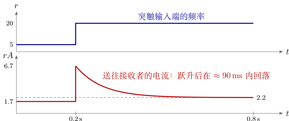
图 4.4: 按公式 (4.6) 工作的压抑型突触, U = 0.5 , \tau_{\text{rec}} = 0.8 s; 电流以每秒 A_0 为单位, 虚线是稳态电流: 它只从 1.7 升到 2.2, 而在跃变瞬间达到 6.7。突触告诉接收者的是频率变了, 而不是频率是多少。
