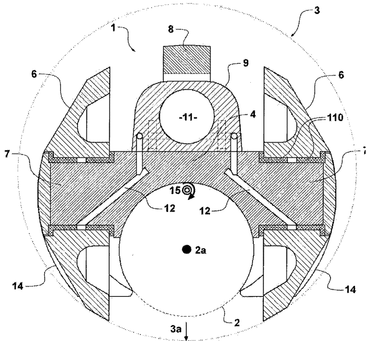
截面A-A
