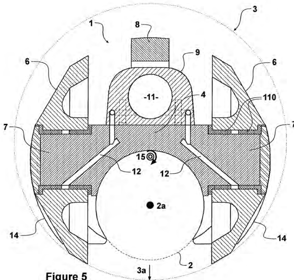
Section A-A
