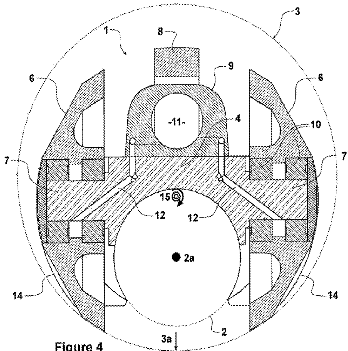
Section A-A
