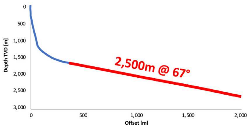
Fig.1. Well Trajectory
