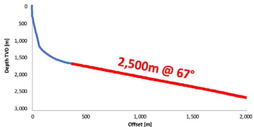
Fig.1. Well Trajectory
