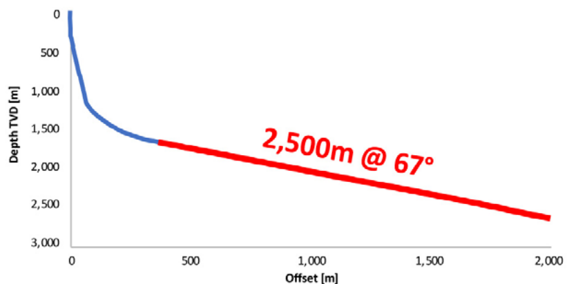
Fig.1. Well Trajectory
