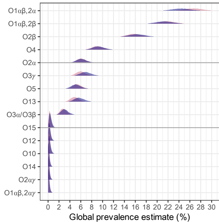
f) Modelled O estimates - posterior
