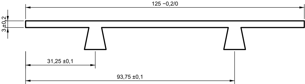
Abschlussblende – Draufsicht (1:1)
