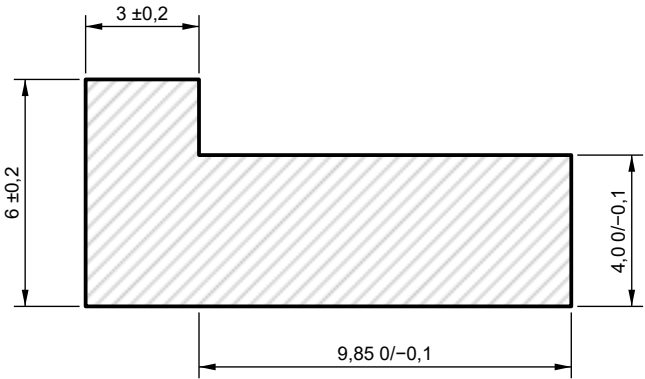
Abschlussblende – Schnitt durch Zunge (5:1)
