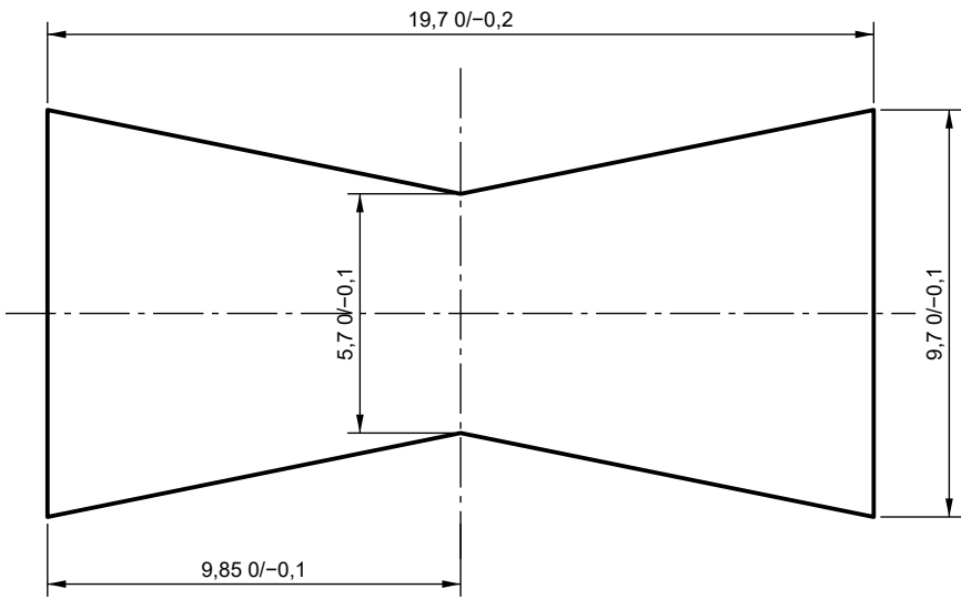
Verbinder – Draufsicht (5:1)
