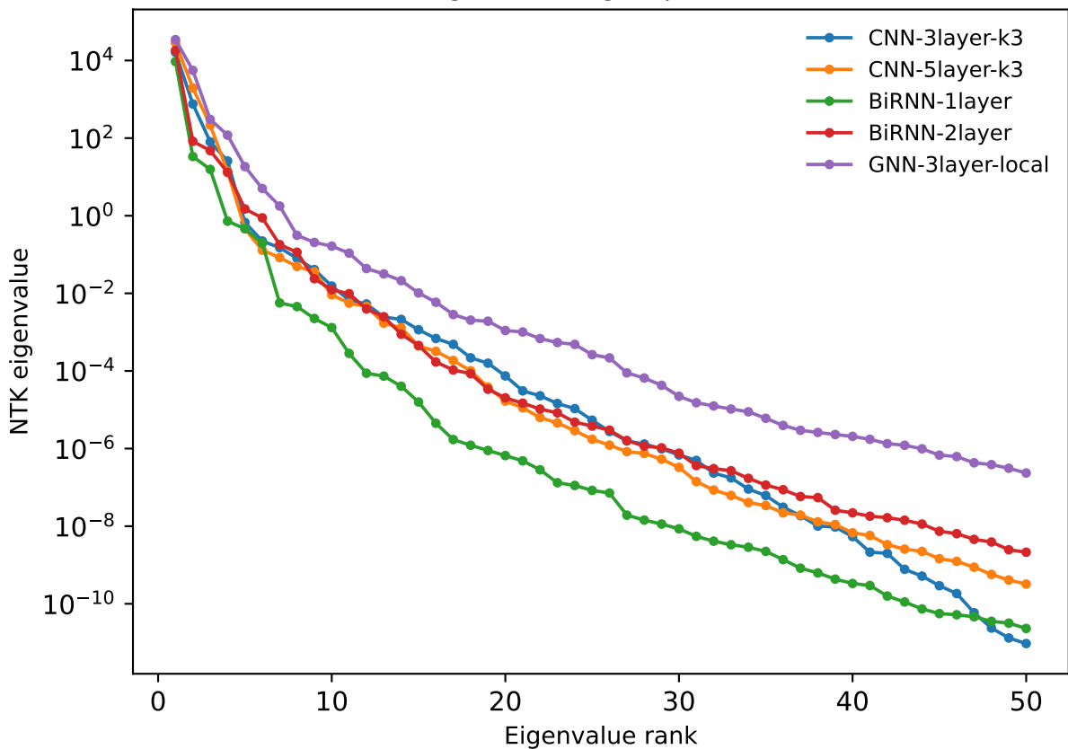
Fig 3 - NTK eigenspectrum
