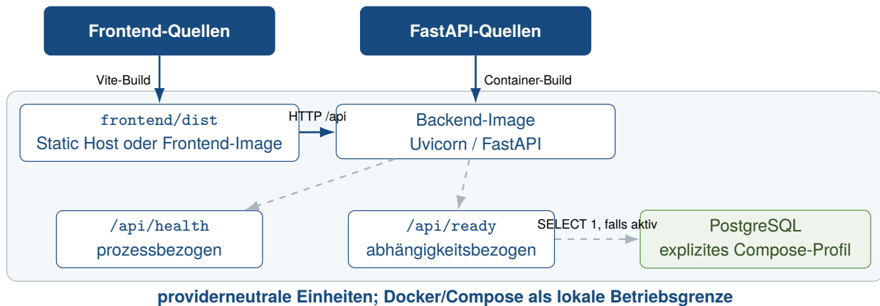
Abbildung 5: Providerneutrale Deployment-Architektur
