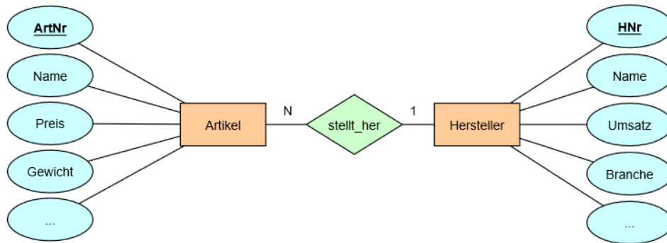
Abb. 3: ER-Diagramm
