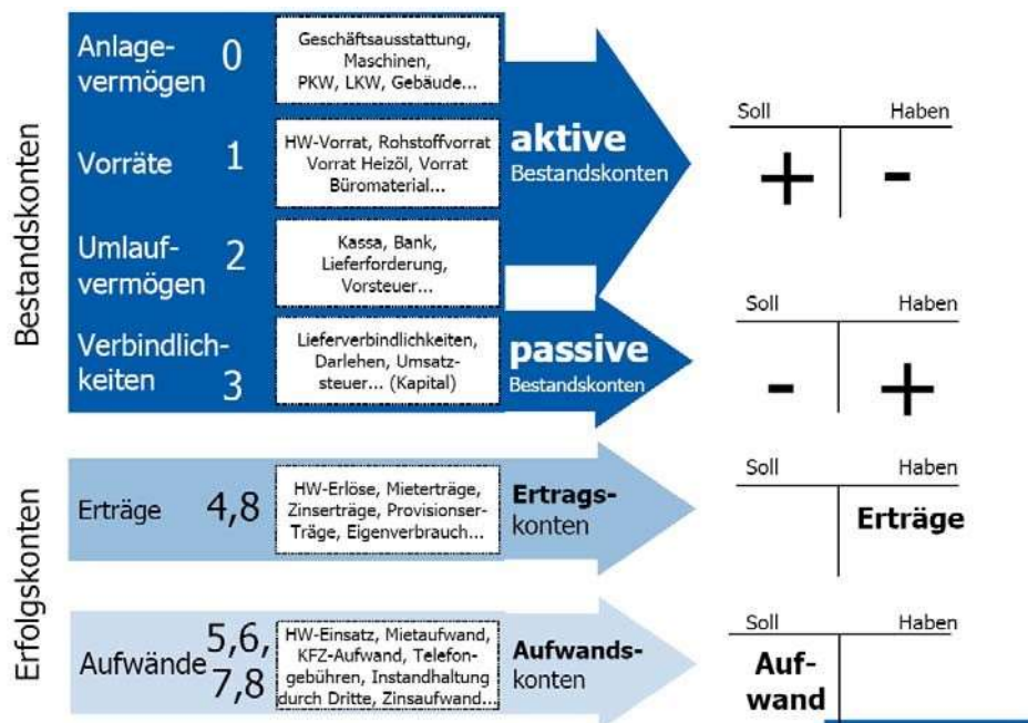
Abb. 16 - Buchungsregeln
