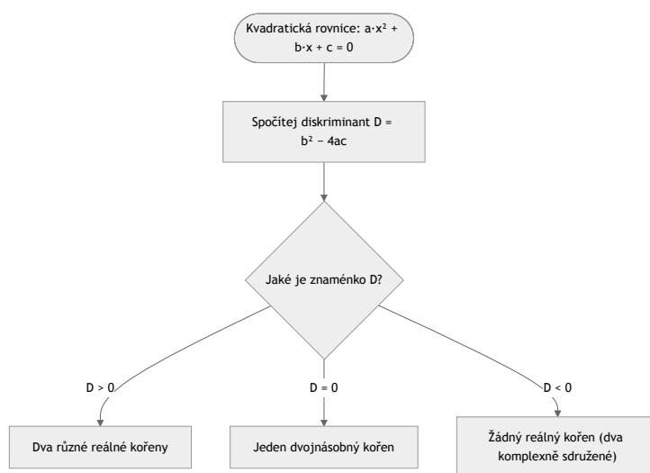
Obrázek 3.2: Vývojový diagram: řešení kvadratické rovnice podle znaménka diskriminantu (Mermaid flowchart).
