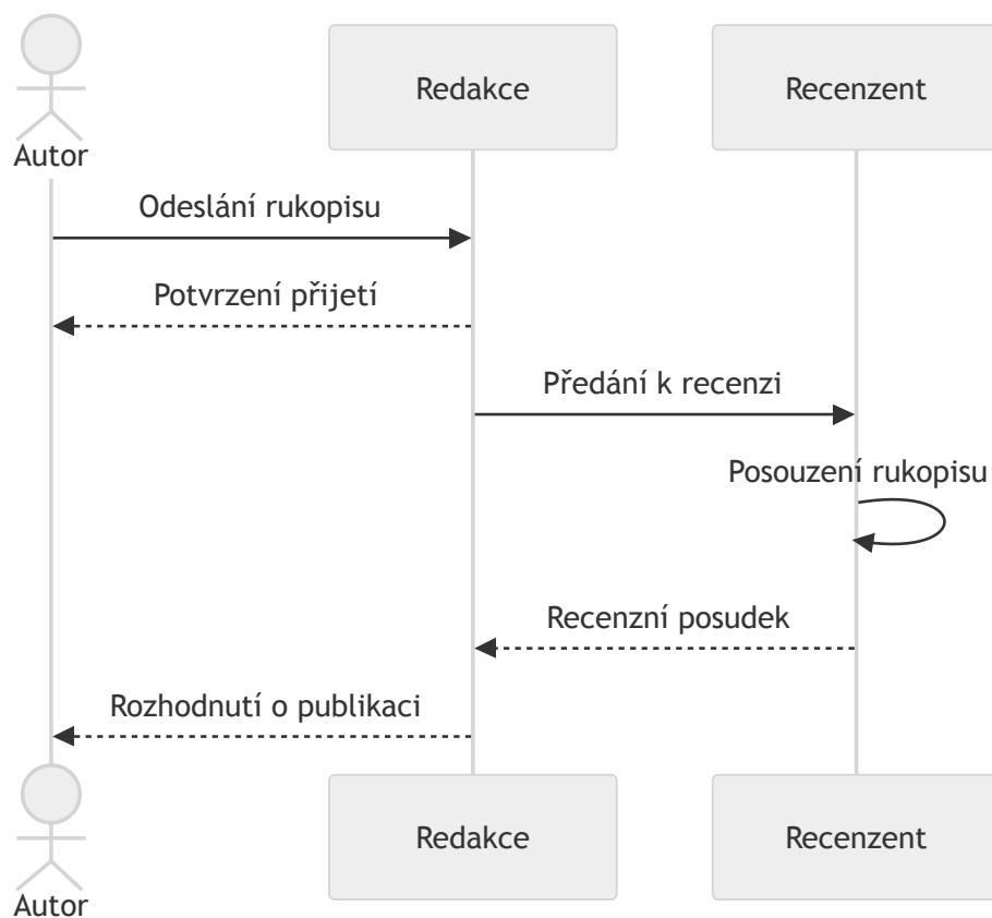
Obrázek 3.3: Sekvenční diagram recenzního řízení rukopisu (Mermaid sequenceDiagram).
