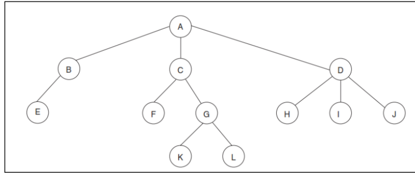
Figura 15.1: Ejemplo de arbol
