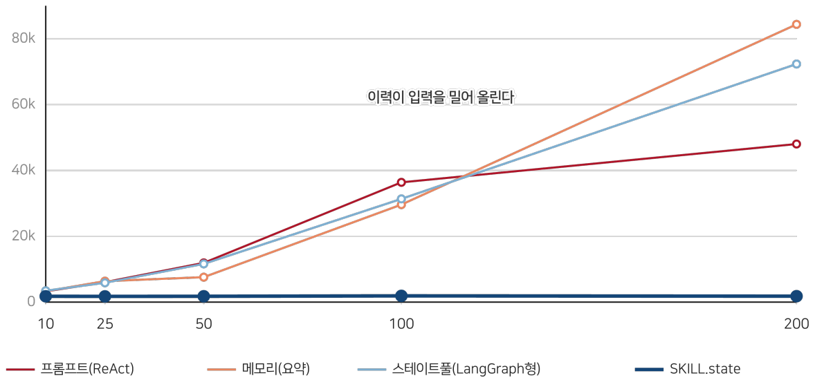
그림 7: 그림 6-2 평균 프롬프트 크기 — SKILL.state는 지평과 무관하게 평평하다
