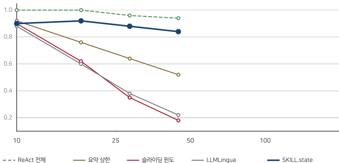
그림 13: 그림 9-2 예산 매칭 스케일링 — 지평이 길어질수록 벌어지는 격차
