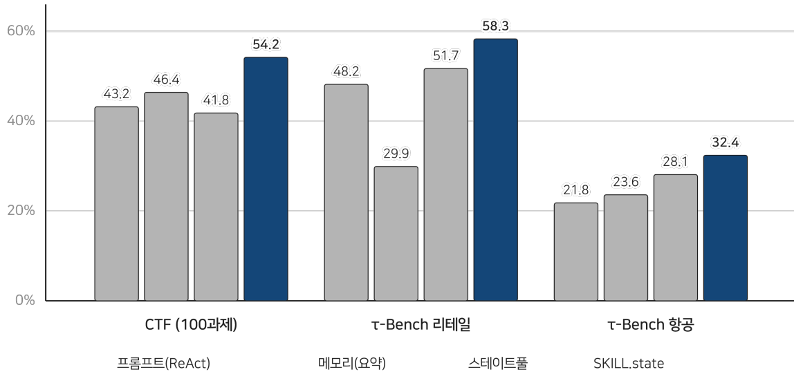
그림 11: 그림 8-1 공개 벤치마크 패스율 — 세 경기 모두 최상위
