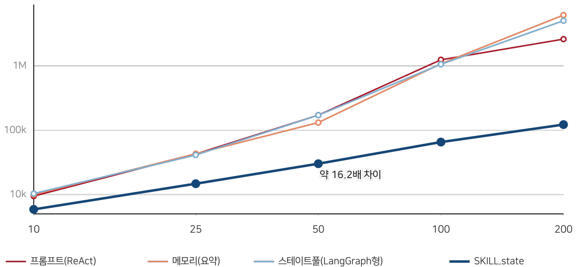
그림 6: 그림 6-1 누적 토큰 소비 — 로그 축 위의 제공 곡선과 선형 직선
