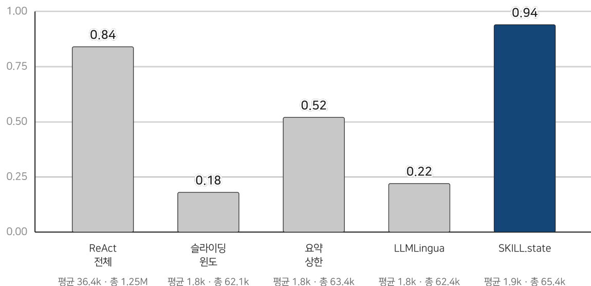
그림 12: 그림 9-1 같은 예산, 다른 결말 — 예산 매칭 대조
