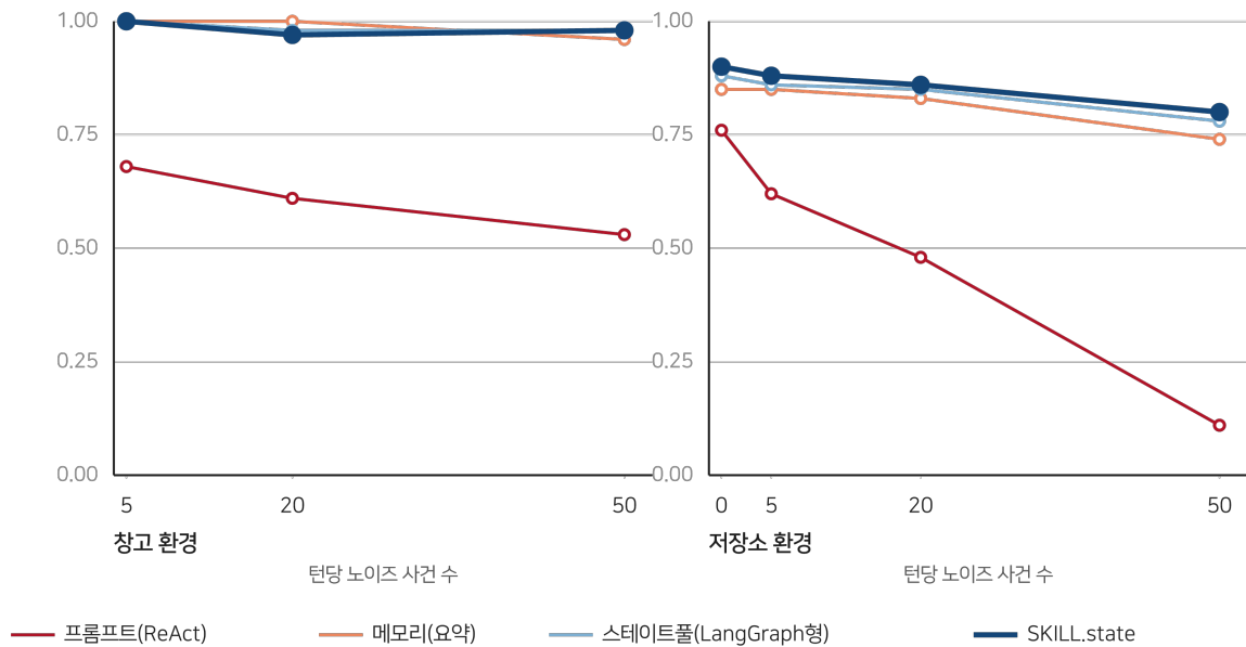
그림 9: 그림 7-1 노이즈 강건성 — 두 환경에서 무너지는 이력, 유지되는 상태
