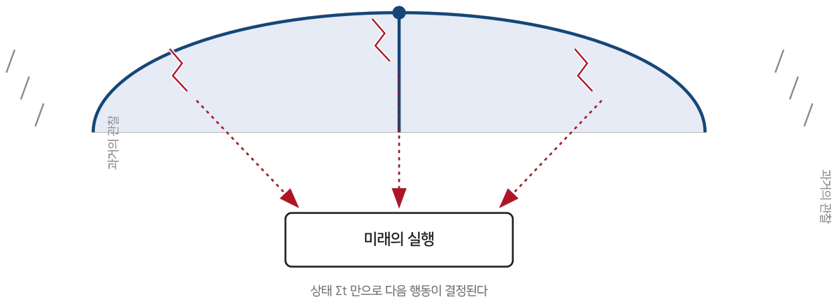
그림 19: 그림 16-1 충분통계량의 우산 — 전제가 깨지는 세 균열
