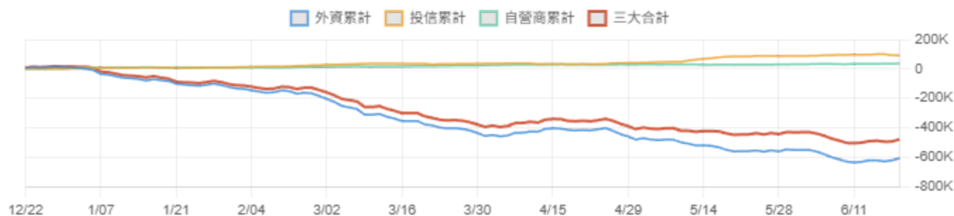
三大法人累計買賣超 (張)
