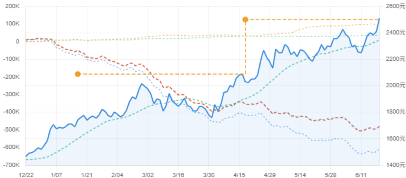
股價走勢 (含三大法人累計買賣超)
