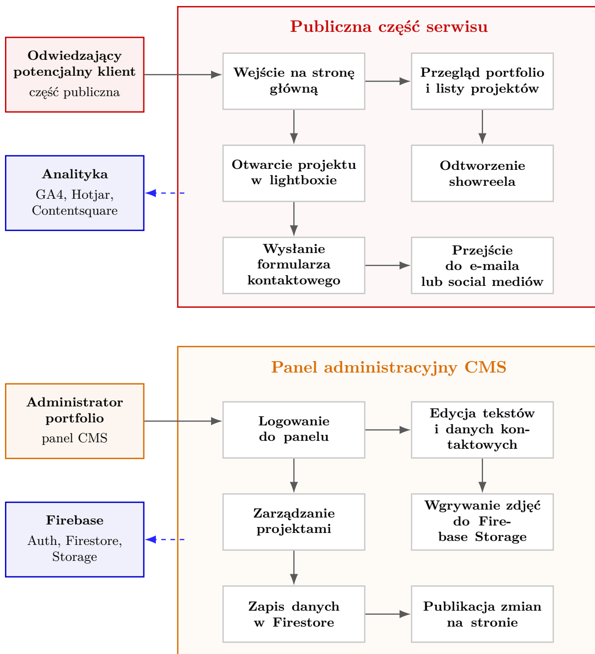
Rysunek 7.1: Diagram funkcjonalności wdrożonej witryny portfolio.
