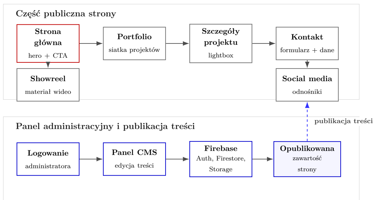
Rysunek 5.1: Schemat architektury informacji serwisu portfolio.
