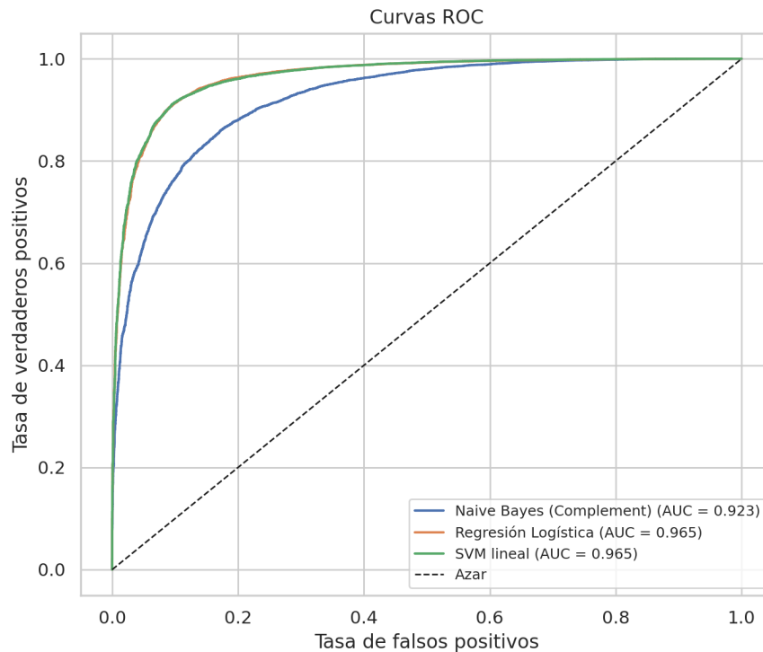
Figura 16: Curvas ROC de los modelos evaluados.
