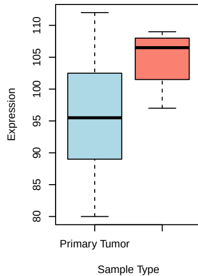
GENE_54
