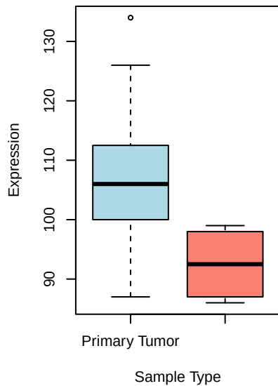
GENE_4
