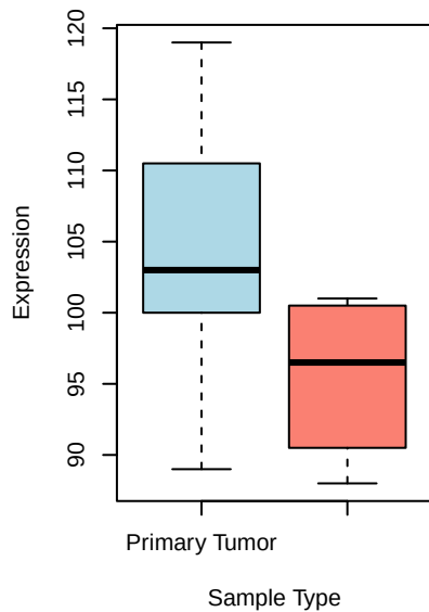
GENE_62
