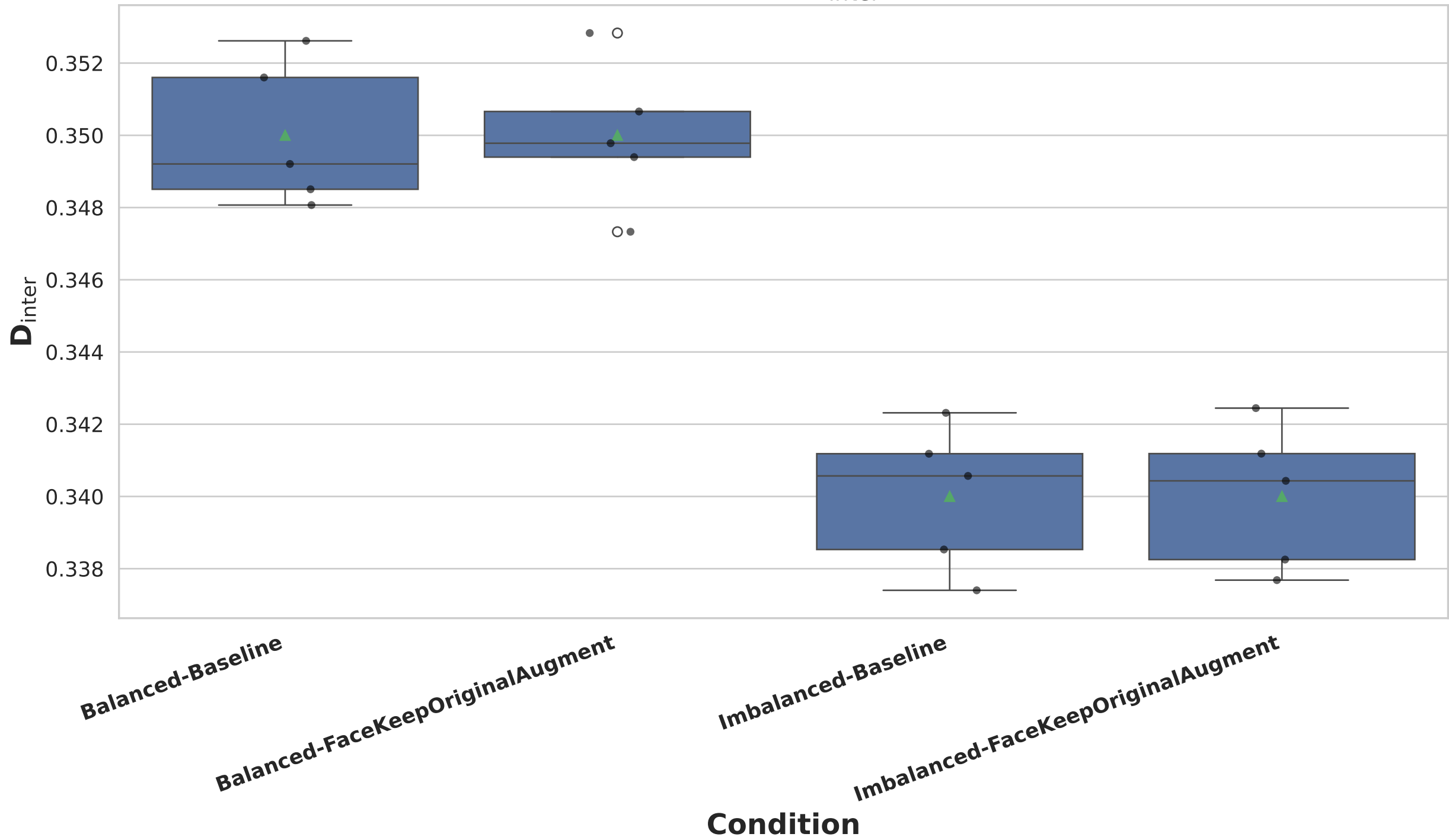
IMDB: D_{inter}
