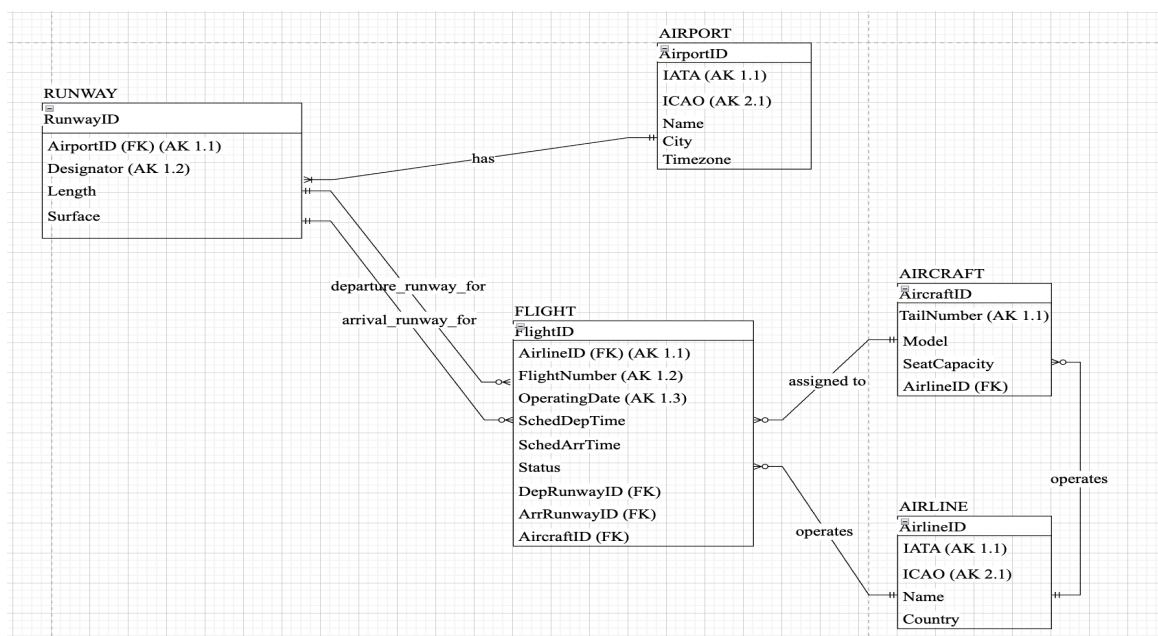
Рисунок 3 – Реляционная модель, полученная из модели
