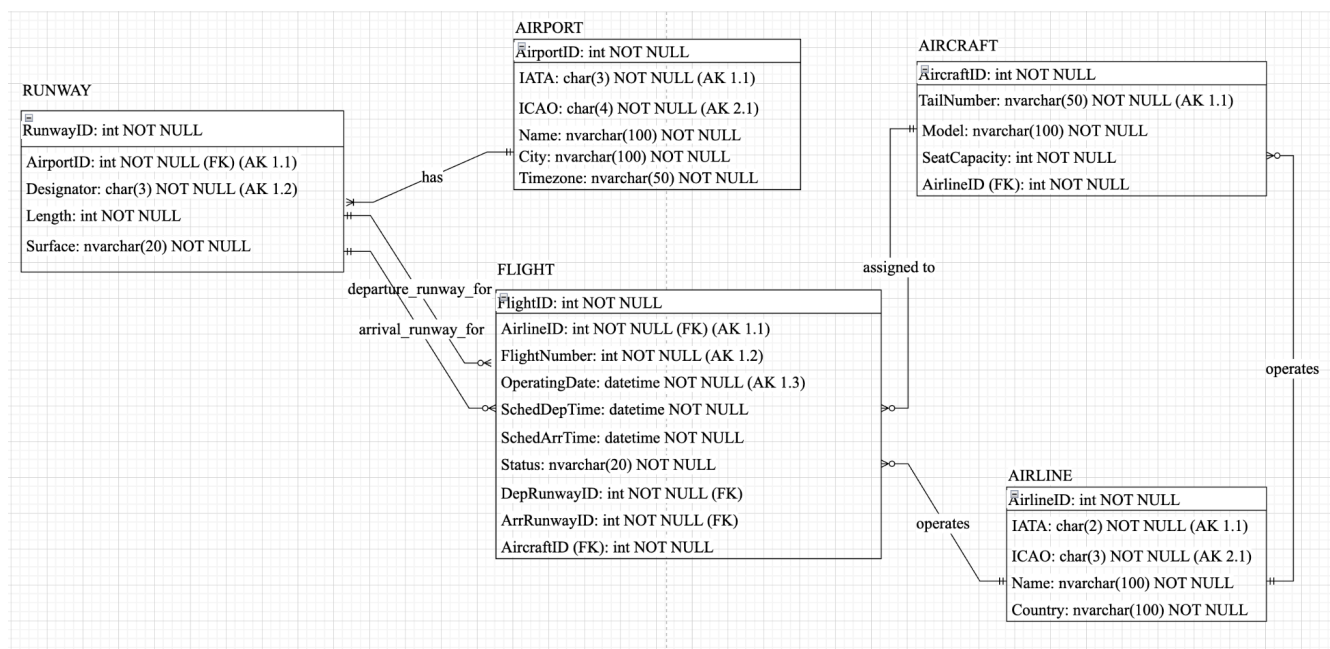
Рисунок 2 – Реляционная модель, полученная из семантических объектов
