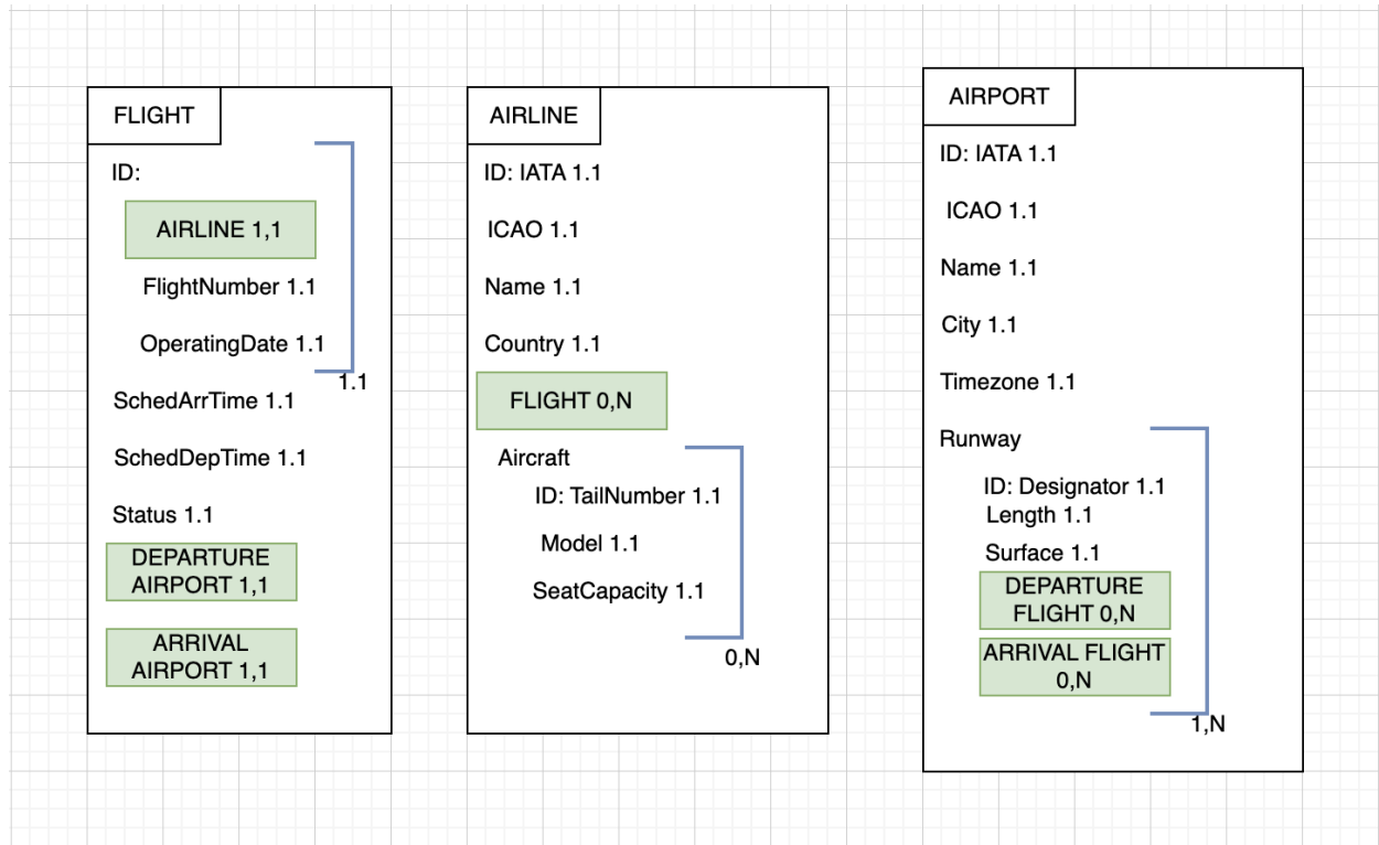
Рисунок 1 – Семантическая объектная модель
