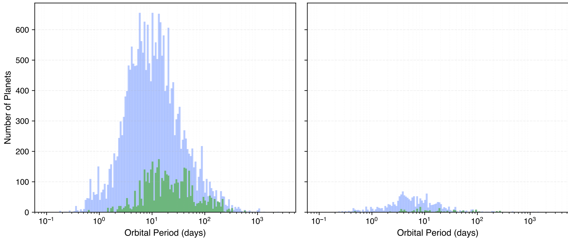
Kepler & K2
