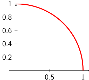
Gambar 2: Segmen lingkaran di kuadran pertama
