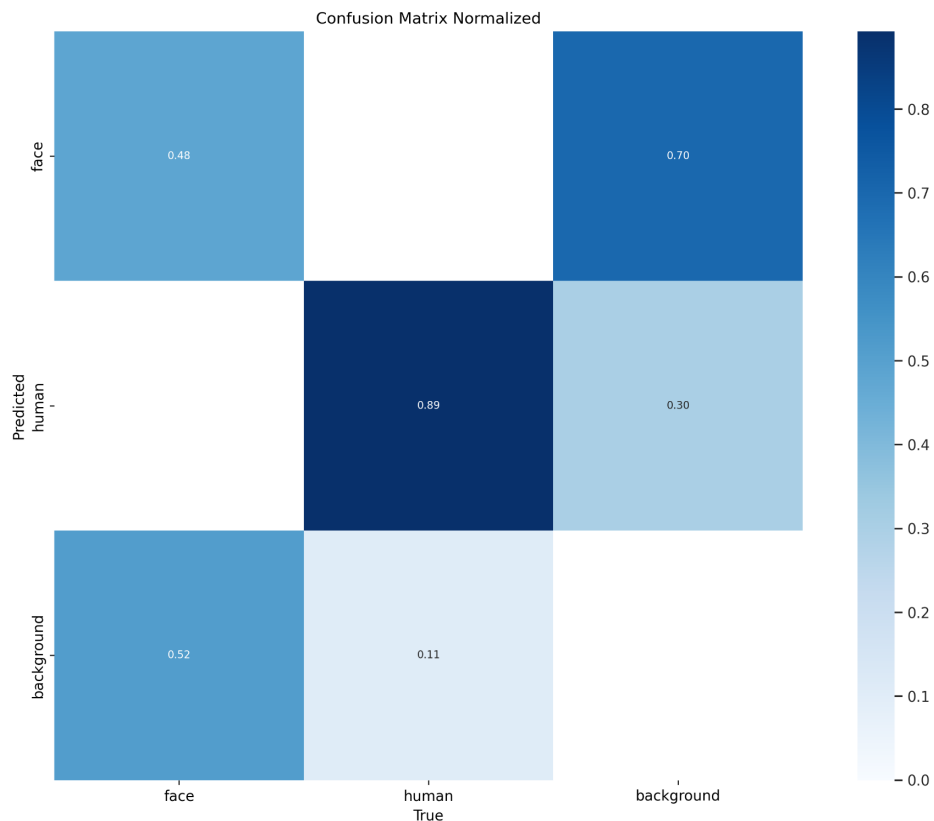
Рисунок 3.2 — Матрица ошибок
