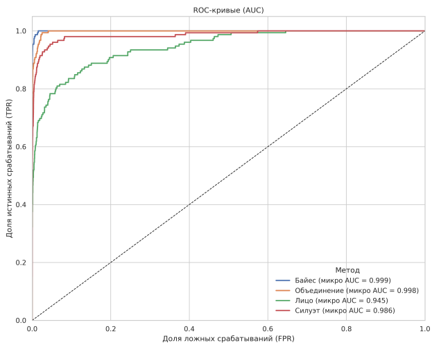
Рисунок 11 – ROC-кривая
