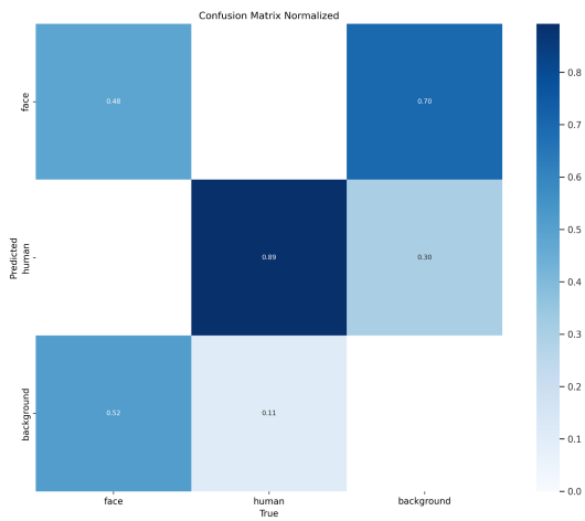
Рисунок 5 – Матрица ошибок
