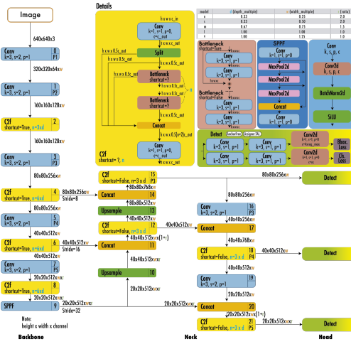
Рисунок 2 – Схема архитектуры YOLOv8
