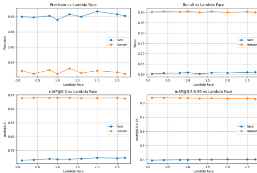
Рисунок 4 – Графики зависимостей показателей качества детекции от \lambda_{\text{face}}
