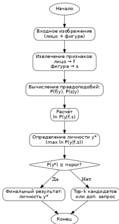
Рисунок 3 – Блок-схема предлагаемого метода байесовской реидентификации
