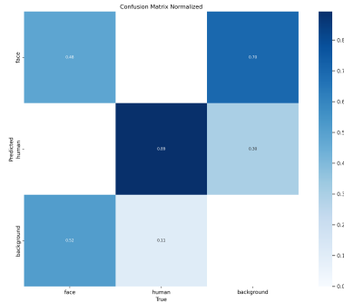
Рисунок 5 – Матрица ошибок
