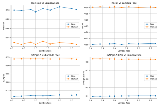
Рисунок 4 – Графики зависимостей показателей качества детекции от \lambda_{\text{face}}
