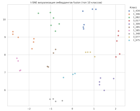
Рисунок 9 – t-SNE для линейного объединения эмбеддингов лица и силуэта
