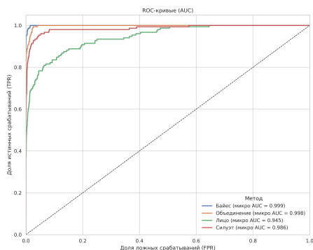
Рисунок 11 – ROC-кривая
