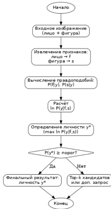
Рисунок 3 – Блок-схема предлагаемого метода байесовской реидентификации
