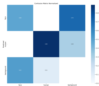
Рисунок 5 – Матрица ошибок
