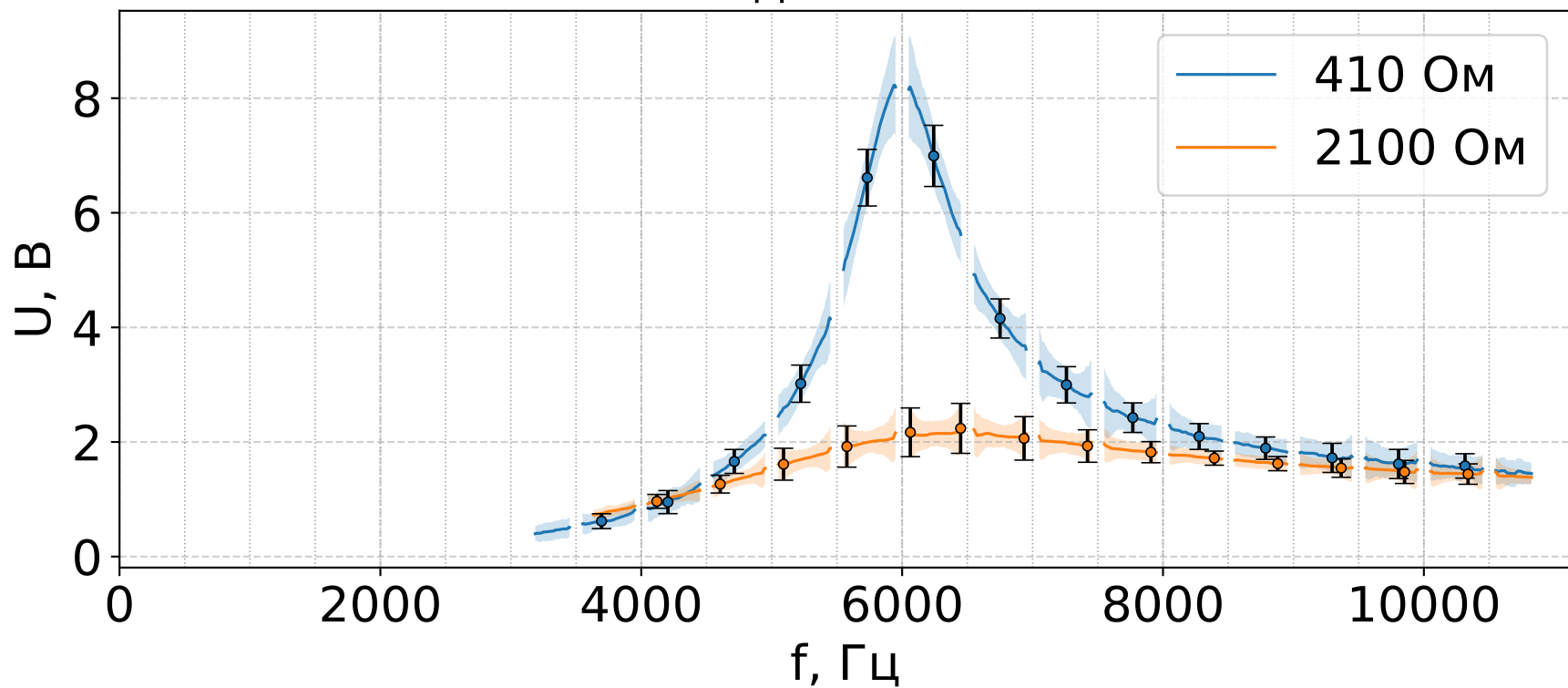
АЧХ для R1 и R2
