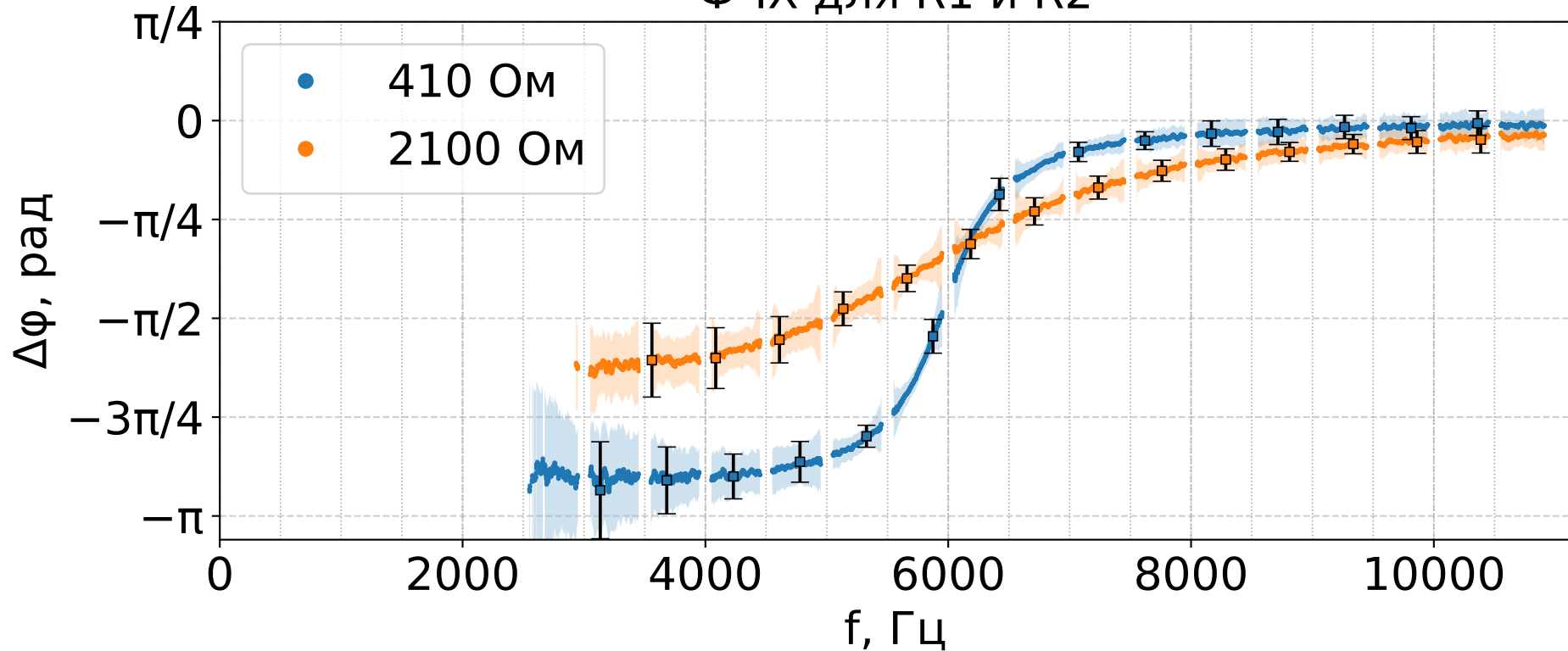
ФЧХ для R1 и R2
