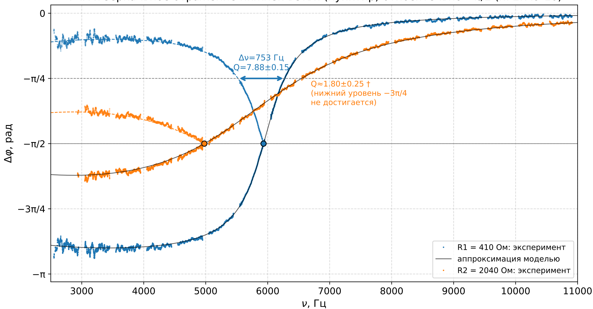
ФЧХ и зеркальное отражение нижней ветви (пунктир) относительно -\pi/2 (п. 2.7.9-10)
