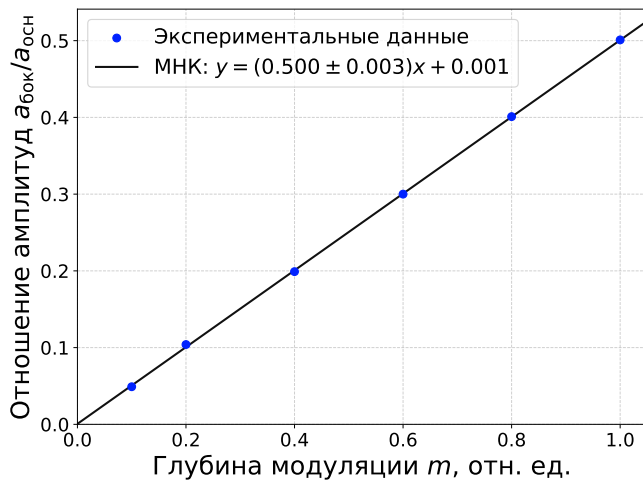
Figure 5. Зависимость отношения амплитуды боковой гармоники к амплитуде основной от глубины модуляции.
