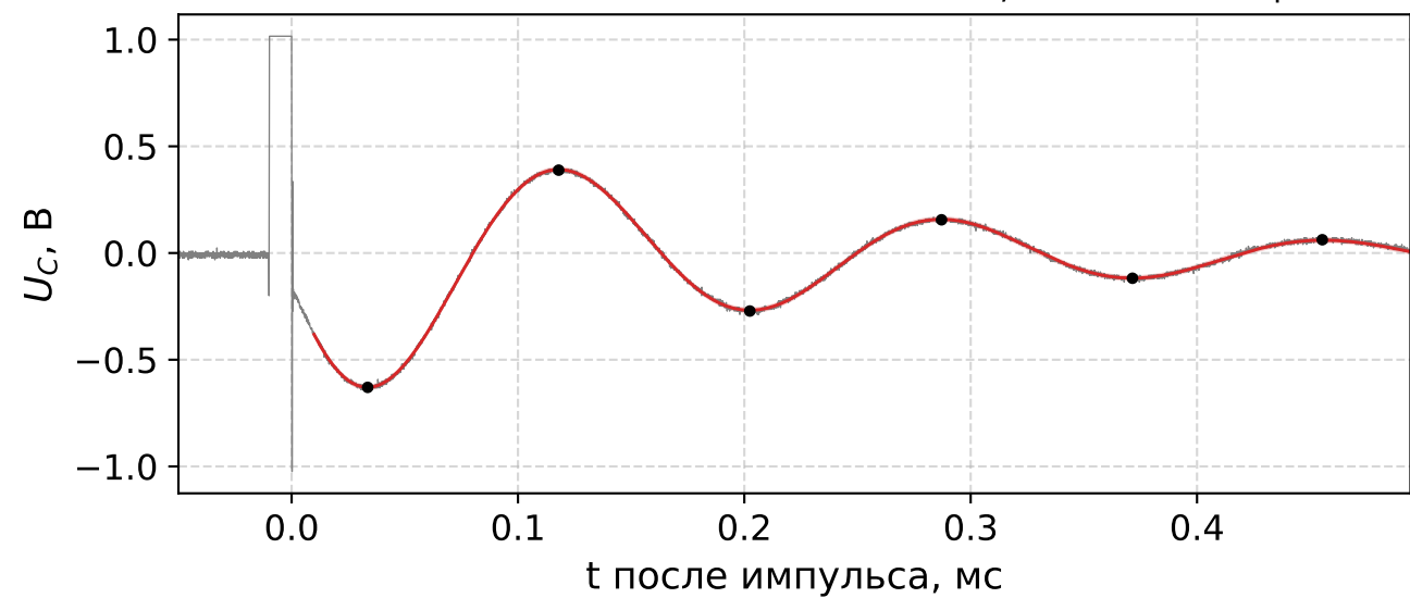
R = 1500 Ом: \Theta = 1.290 \pm 0.008 , f = 5863 Гц
