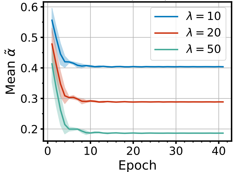
Mean \tilde{\alpha} per Epoch
