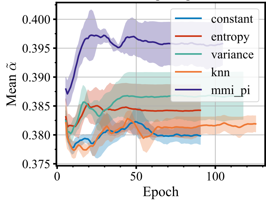
Mean \tilde{\alpha} per Epoch
