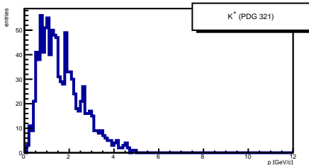
K + momentum
