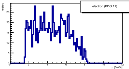
e' momentum
