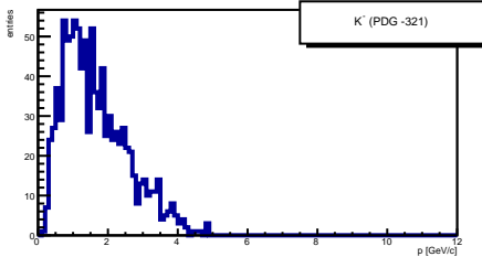
K - momentum
