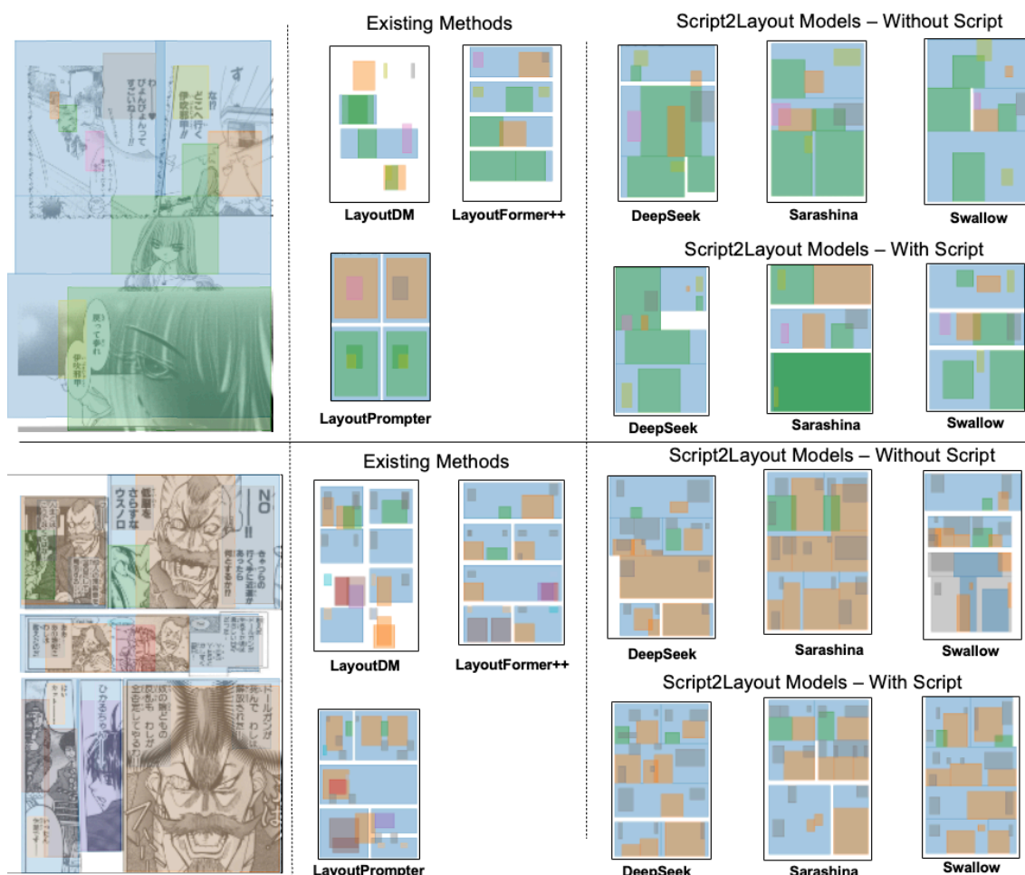
図 1.2: Gen-T 条件下におけるレイアウト生成の可視化結果. 各行に対して, 左から順に正解レイアウト, 既存手法の生成例, Script2Layout の生成例, が並び, Script2Layout では上段に Script 条件なし, 下段に Script 条件ありの結果を示す. (漫画: 上段『ヒーリング・プラネット』© 桜野 みねね/エニックス, 下段『ドールガン』© 出口 竜正/秋田書店)
