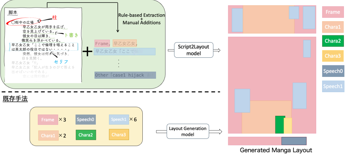
図 1.1: Script2Layout による脚本条件付きレイアウト生成の概略図。上段は、本研究で提案する手法であり、自然言語として記述された脚本を直接入力として扱いつつ、キャラクター、セリフ、およびコマに対応する要素を抽出し、Fine-tuned LLM によりページ全体のレイアウトを生成する。下段は、既存のレイアウト生成手法の例であり、要素数やカテゴリといった構造化情報を入力としてレイアウトを生成する点で異なる。
