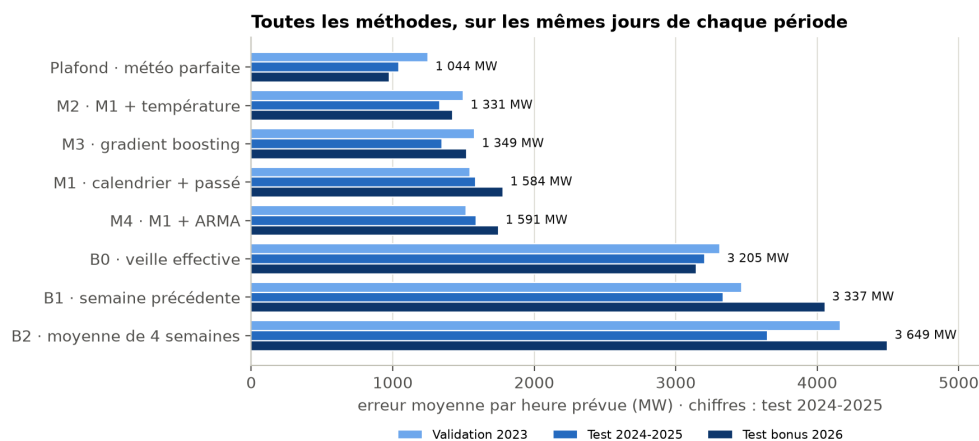
FIGURE 3 – Comparaison des modèles sur validation, test et période complémentaire.
