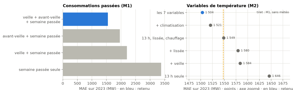
FIGURE 2 – Ablations sur la validation 2023 : contribution des retards et de la météo.
