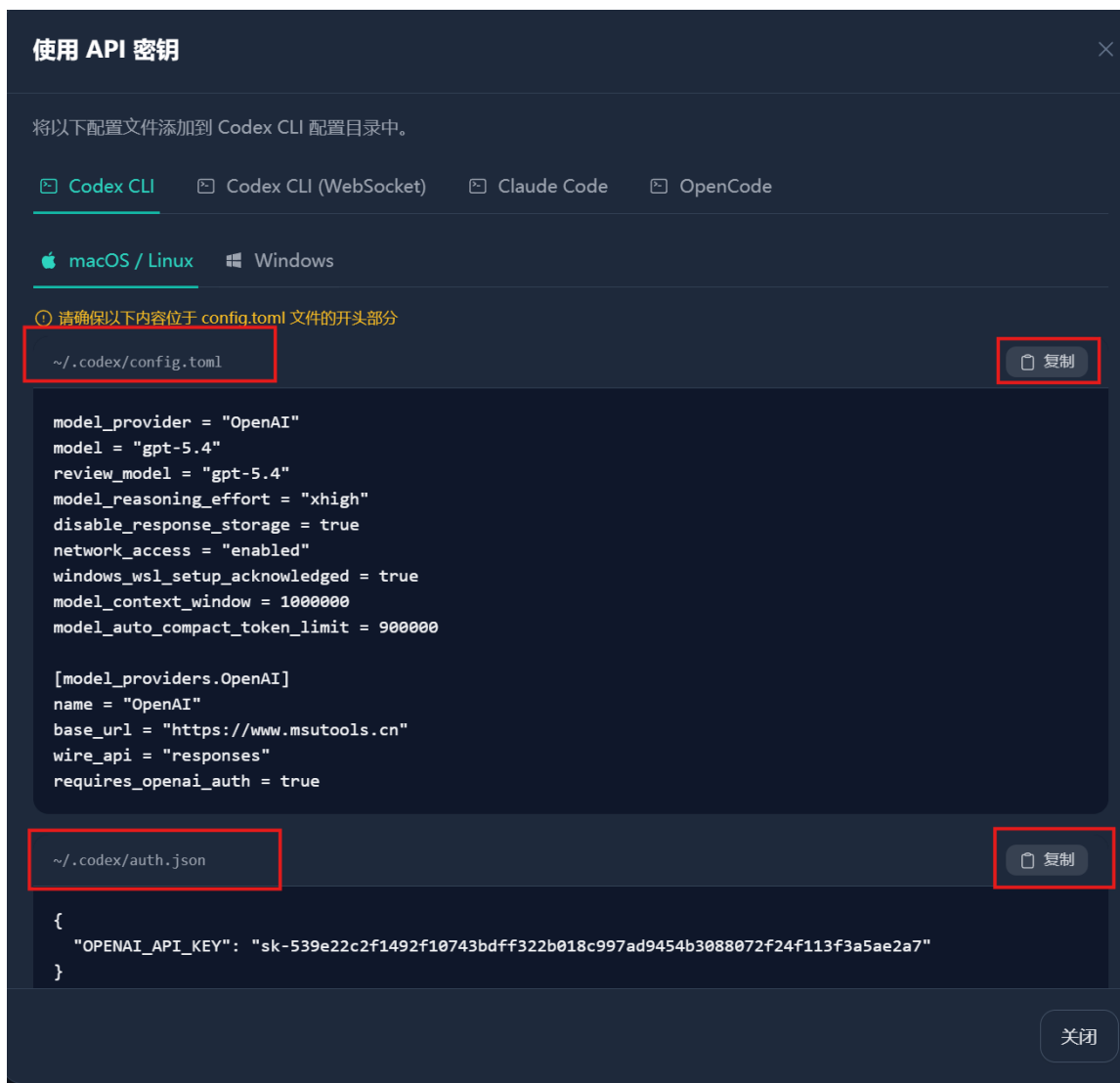
图 5: 复制 API Key 和配置 (分别在登录和配置是复制)
