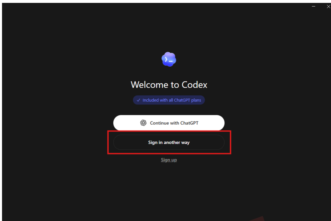
图 6: 登录
