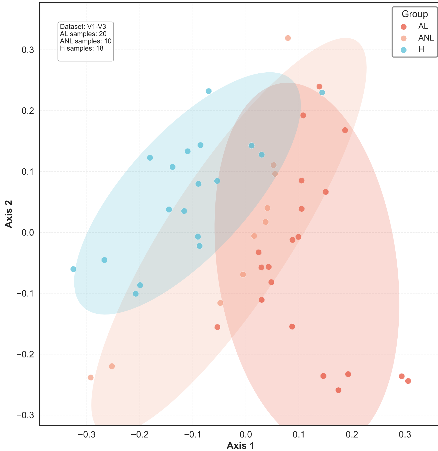
V1-V3 Ordination
