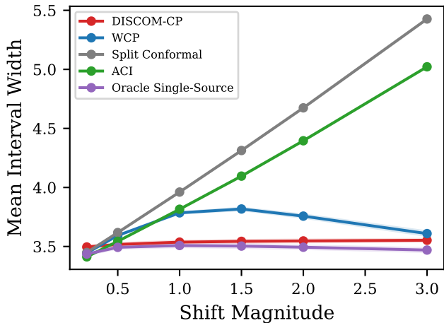
Interval Width vs. Shift Magnitude
