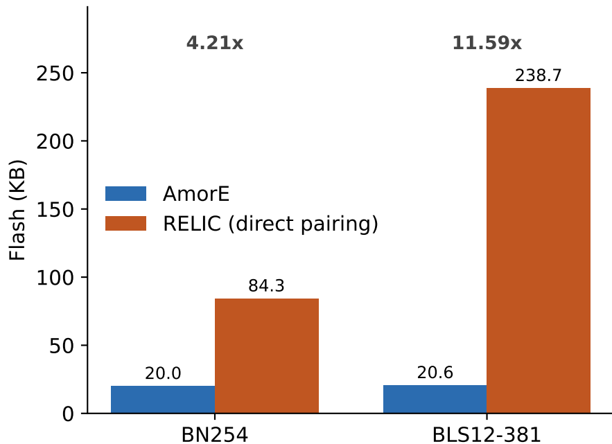
Flash (code+rodata)
