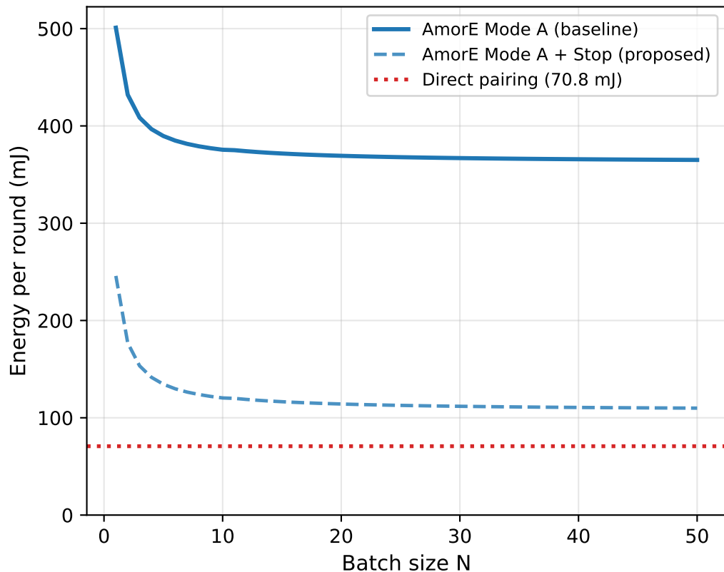
BN254
