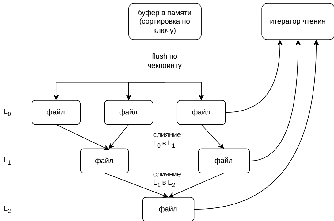
Рисунок 1 — Устройство LSM-дерева бакета в Apache Raïmon: буферизация в памяти, сброс в L_0 по чекпойнту, фоновое слияние на нижележащие уровни, объединение версий итератором слияния при чтении
