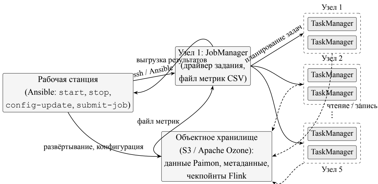
Рисунок 3 – Схема развёртывания окружения нагрузочного тестирования: автоматизация через Ansible, кластер из пяти узлов (по два менеджера задач на узел), объектное хранилище как бэкенд данных и чекпойнтов
