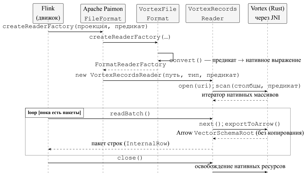
Рисунок 2 – Диаграмма последовательности: чтение таблицы Apache Paimon с файловым форматом Vortex
