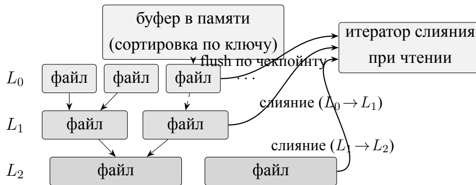
Рисунок 1 – Устройство LSM-дерева бакета в Apache Raimon: буферизация в памяти, сброс в L_0 по чекпойнту, фоновое слияние на нижележащие уровни, объединение версий итератором слияния при чтении
