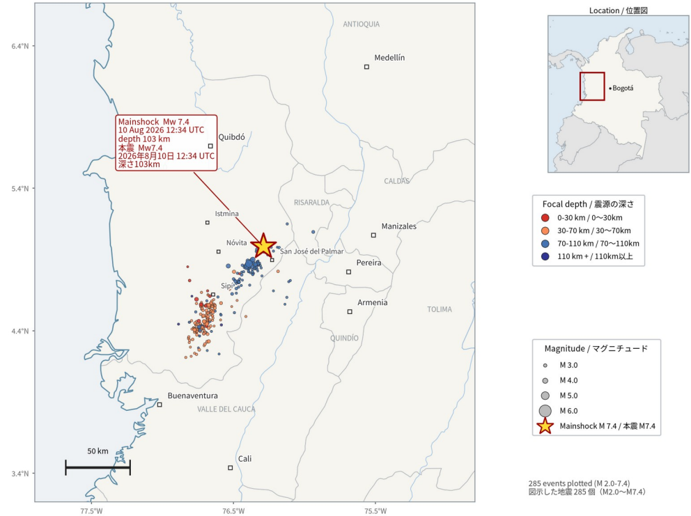
2026 Chocó Earthquake (Colombia) — Epicentre distribution 2026年コロンビア・チョコ地震 震央分布図 Mainshock and aftershocks, 10-19 August 2026 本震および余震 (2026年8月10日～19日)
